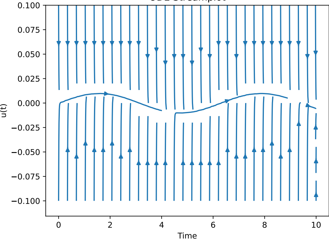
ODE Streamplot
