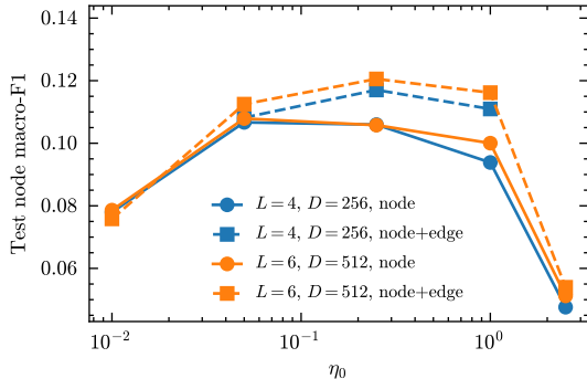
CPEN
