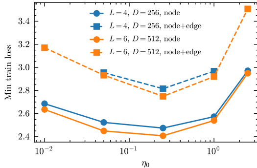
CPEN
