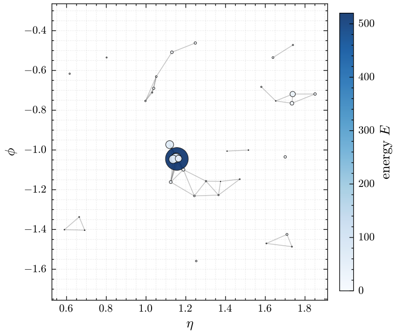
QCD jet 49390
