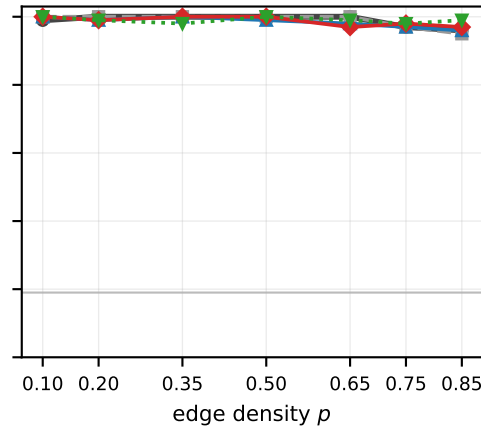
qwen3-4b-think
