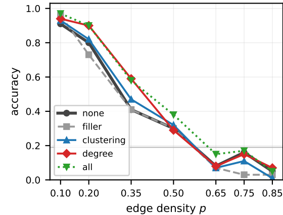
qwen3-1.7b
