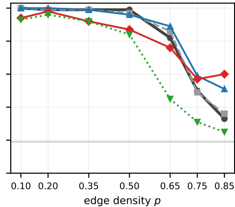
qwen3-4b
