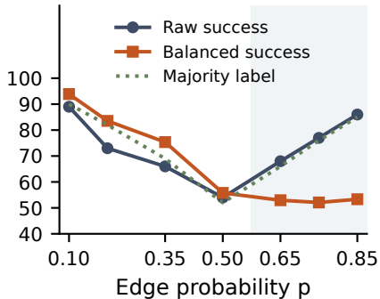
(b) 1.7B: edge existence
