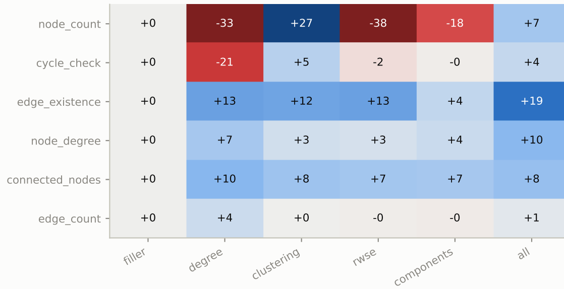
qwen3-1.7b
