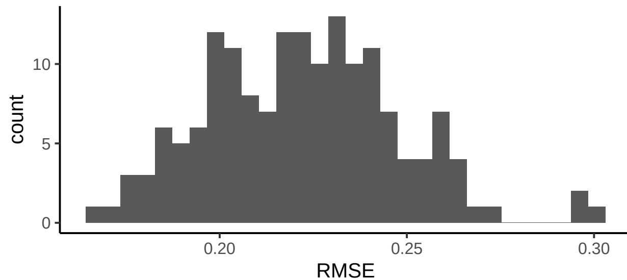
Adults: EIG
