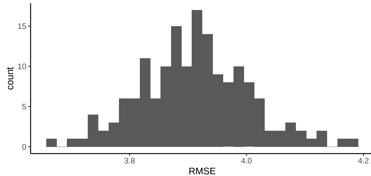
KL
