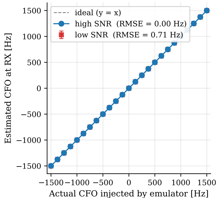
(a) Estimated vs actual CFO
