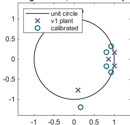
Eigenvalues, 50 Hz AFC loop
