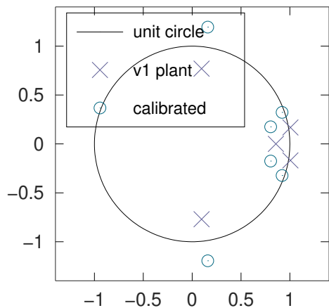
Eigenvalues, 50 Hz AFC loop
