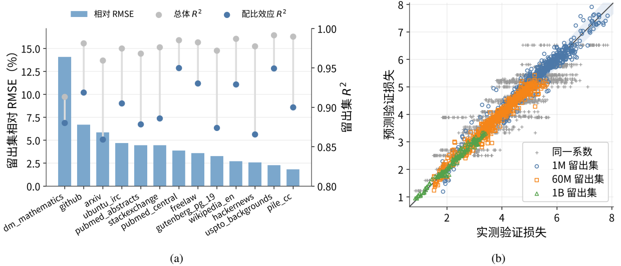
图 5.9 广义标度律的留出配比较验证：(a) 各评估目标的相对 RMSE、总体 R^2 与配比效应 R^2 ；(b) 三个观测规模的实测与预测损失对比，灰色标记为同一组系数下关闭配比项的预测，实线为理想一致线，阴影表示 \pm 5\% 误差带。
