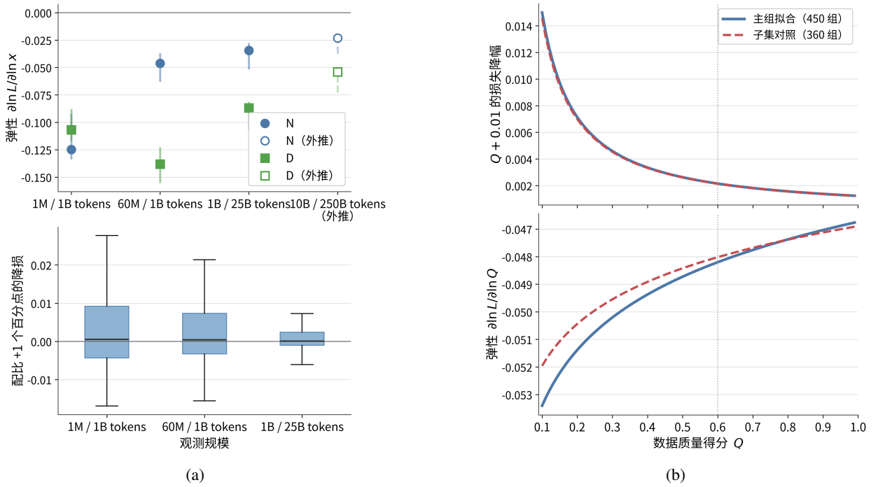
图 5.10 资源与质量因素的局部响应：(a) 参数量和数量数据的损失弹性，以及配比份额增加 1 个百分点的方向收益分布；区间表示跨评估目标的四分位范围，百亿参数点仅为外推。(b) 独立质量实验中质量分增加 0.01 的降损及损失弹性；对照组为主组子集。
