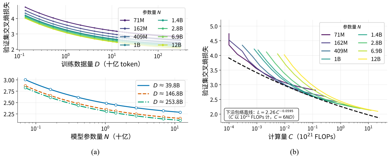
图 10.6 经典标度律的资源标度与计算效率：(a) 参数规模、数据规模与验证损失的标度关系；(b) 不同参数规模下计算量与验证损失的关系，虚线为经验下沿包络。
