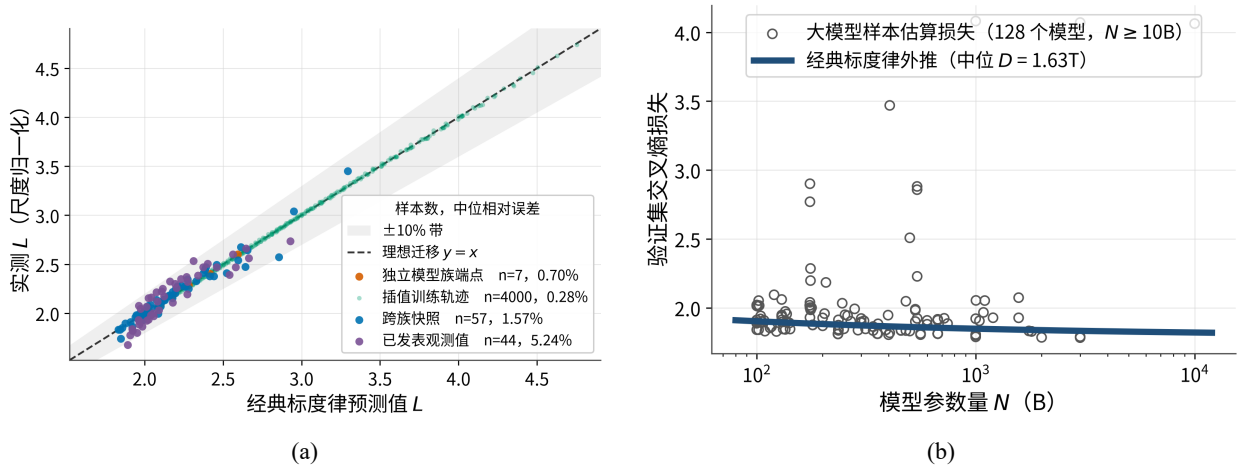
图 10.7 经典标度律的跨来源验证与大模型外推：(a) 损失尺度归一化后的多来源预测一致性，虚线为理想预测，阴影区域表示相对误差不超过 10%；(b) 百亿参数以上模型区间的标度律外推，曲线按中位训练数据量计算。
