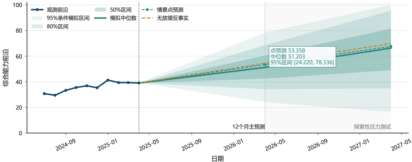
算力平台情景下的能力前沿预测
