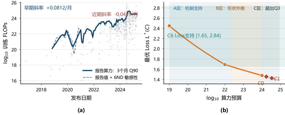
图 7.4 训练算力演进与 Q3–C6 共同支持边界
