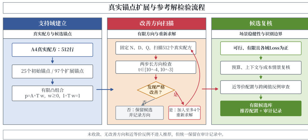
图 6.18 真实锚点扩展与参考解检验流程
