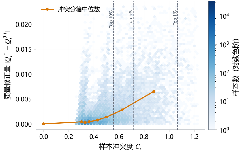
图 4.4 冲突修正的局部性与异常来源
