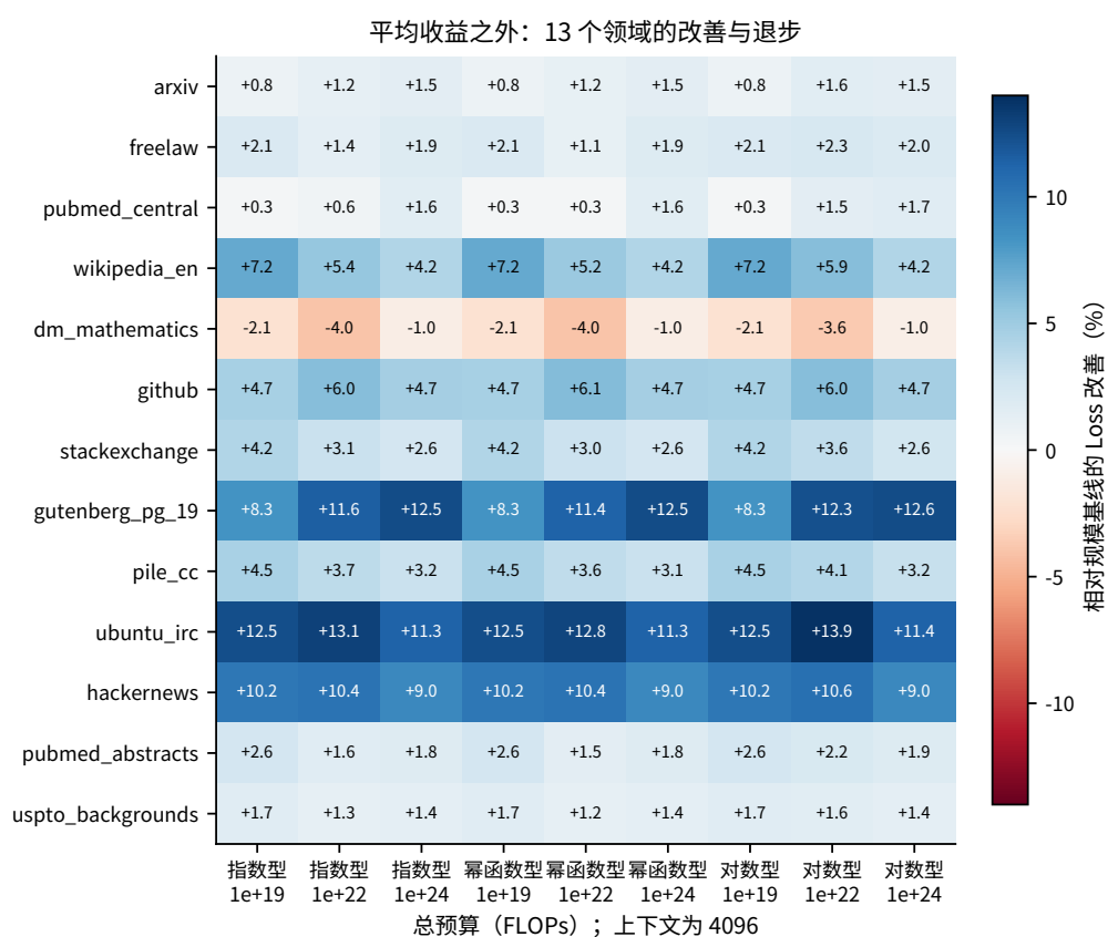
图 6.20 典型配置的逐域代价；热力图保留 13 个评测域和 9 组预算-成本组合，颜色表示相对原配方的 Loss 变化
