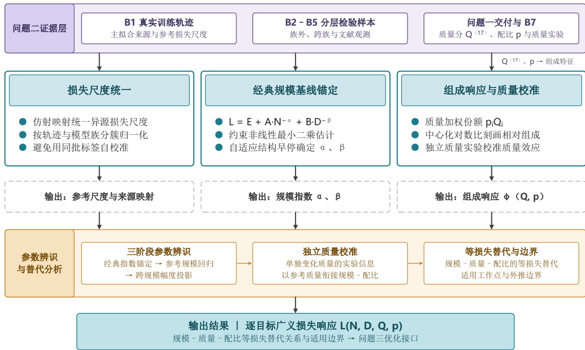
图 5.7 问题二的整体分析框架：经典规模基线及跨来源检验、质量与配比的广义律构造，以及边际响应和等损失替代分析。
