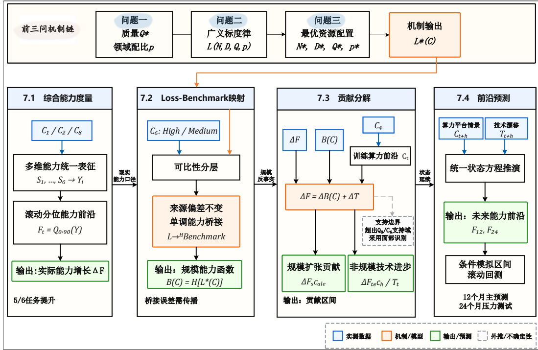
图 7.1 前三问机制输出与能力前沿分析的统一框架
