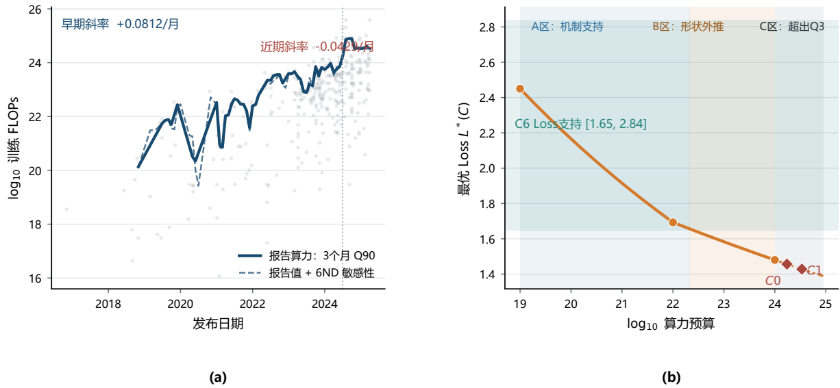
图 7.4 训练算力演进与 Q3–C6 共同支持边界。(a) 报告训练算力的滚动前沿与敏感性曲线。(b) Q3 最优损失曲线、C6 桥接范围及域外层级
