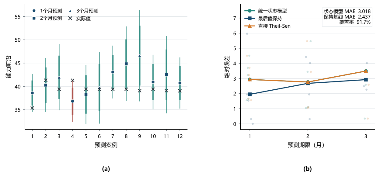
图 7.8 能力前沿预测的滚动起点回测与简单基线比较。(a) 统一状态模型的逐案例区间预测。(b) 三类方法在不同预测期限下的绝对误差
