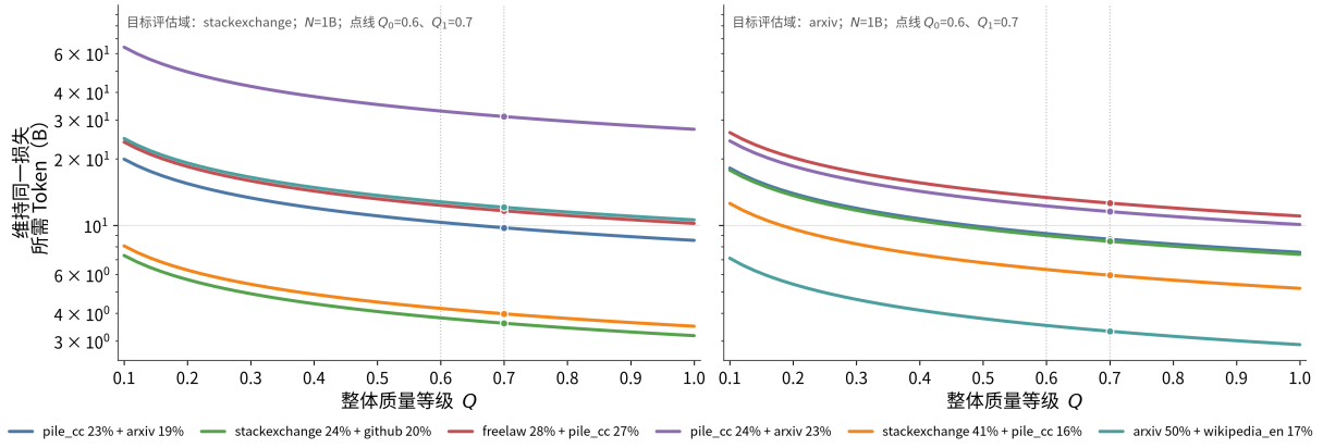
图 5.14 两种示例评估领域的质量—Token 等损失曲线。各曲线对应同一组观测配比，纵轴为保持参考目标损失所需的 Token 数； Q_0 = 0.6 与 Q_1 = 0.7 为质量比较点。离开 N = 10^9 , D_\star = 250 亿 Token 观测工作点后的需求量属于模型情景推算。
