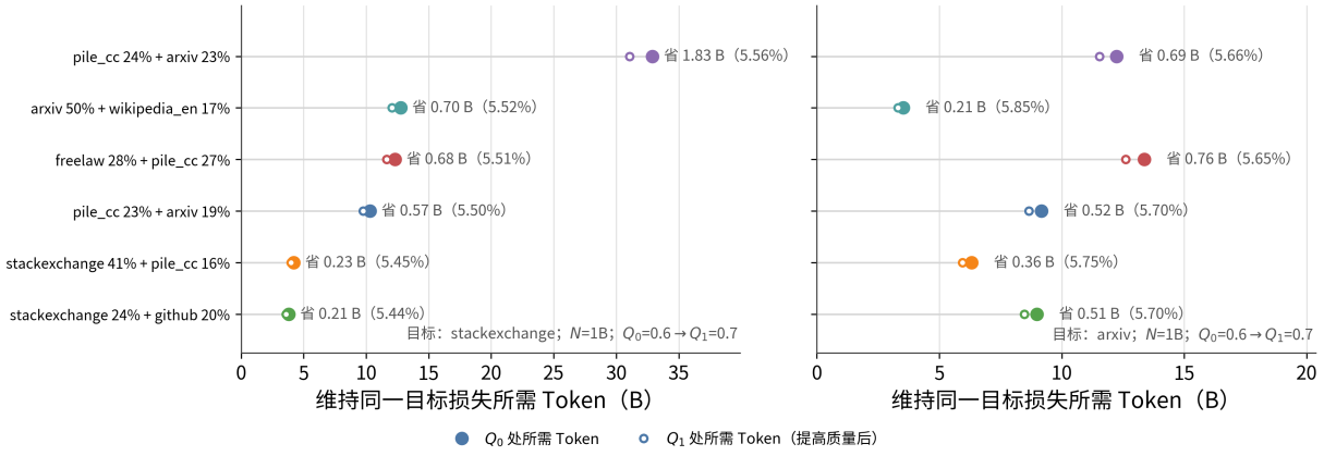
图 5.15 同一组观测配比在两种示例评估领域中的等损失 Token 需求。各行配比保持一致，实心与空心标记分别对应 Q_0 = 0.6 和 Q_1 = 0.7 ；横向差异表征模型预测的配比依赖性，并非配比干预的因果效应。
