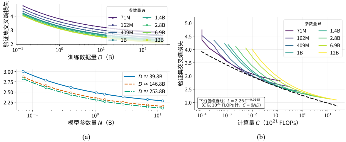
图 5.9 经典标度律的资源标度与计算效率：(a) 参数规模、数据规模与验证损失的标度关系。(b) 不同参数规模下计算量与验证损失的关系，虚线为经验下沿包络。
