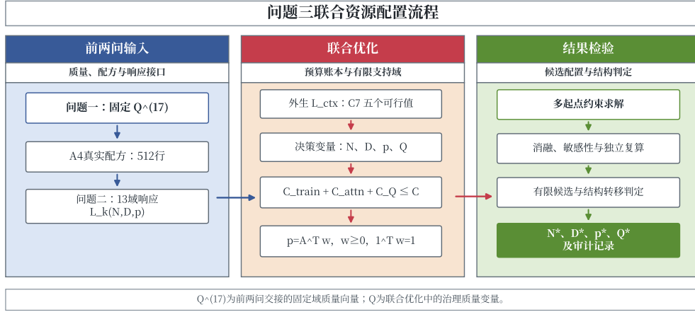
图 6.16 质量、配方及规模响应的衔接与联合求解流程
