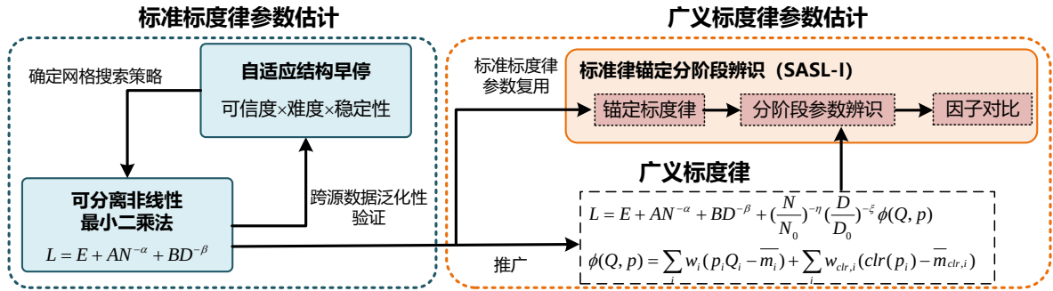
图 5.8 广义标度律的三阶段参数辨识：标准律锚定规模指数，分阶段估计组成响应与基线，再由规模因子对比确定响应幅度指数。
