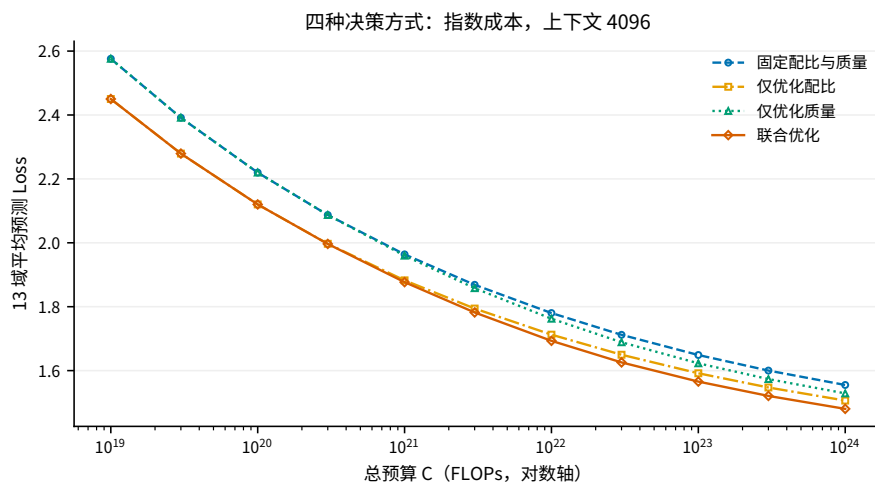
图 6.19 指数成本、上下文 4096 时 11 档预算的四组消融：各组均联动优化 N/D
