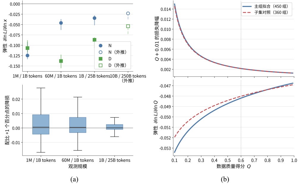
图 5.12 资源与质量因素的局部响应：(a) 参数量和数据量的损失弹性，以及配比份额增加 1 个百分点的方向收益分布；区间表示跨评估目标的四分位范围，百亿参数点仅为外推。(b) 独立质量实验中质量分增加 0.01 的降损及损失弹性；对照组为主组子集。
