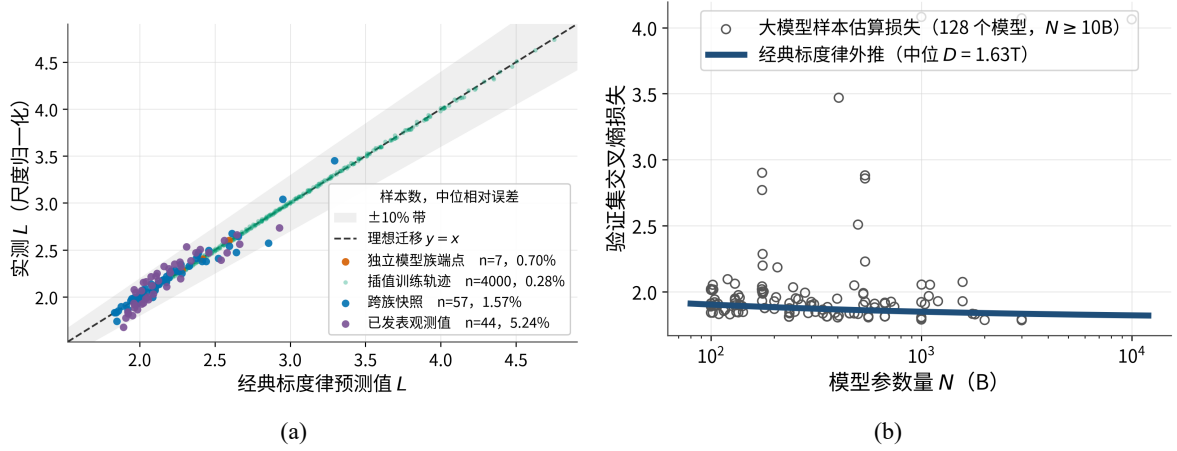
图 5.10 经典标度律的跨来源验证与大模型外推：(a) 损失尺度归一化后的多来源预测一致性，虚线为理想预测，阴影区域表示相对误差不超过 10%；(b) 百亿参数以上模型区间的标度律外推，曲线按中位训练数据量计算。
