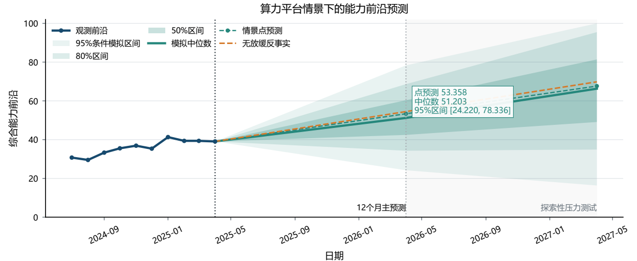
图 7.6 算力平台情景下开放权重模型能力前沿的条件预测
