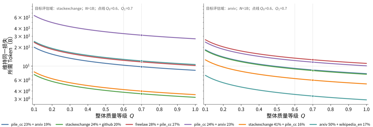
图 5.8 两种示例评估领域的质量-Token 等损失曲线。各曲线对应同一组观测配比, 纵轴为保持参考目标损失所需的 Token 数; Q_0 = 0.6 与 Q_1 = 0.7 为质量比较点。离开 N = 10^9 , D_\star = 250 亿 Token 观测工作点后的需求量属于模型情景推算。
