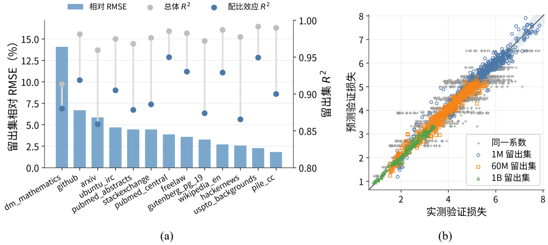
图 5.10 广义标度律的留出配比验证：(a) 各评估目标的相对 RMSE、总体 R^2 与配比效应 R^2 ；(b) 三个观测规模的实测与预测损失对比，灰色标记为同一组系数下关闭配比项的预测，实线为理想一致线，阴影表示 \pm 5\% 误差带。
