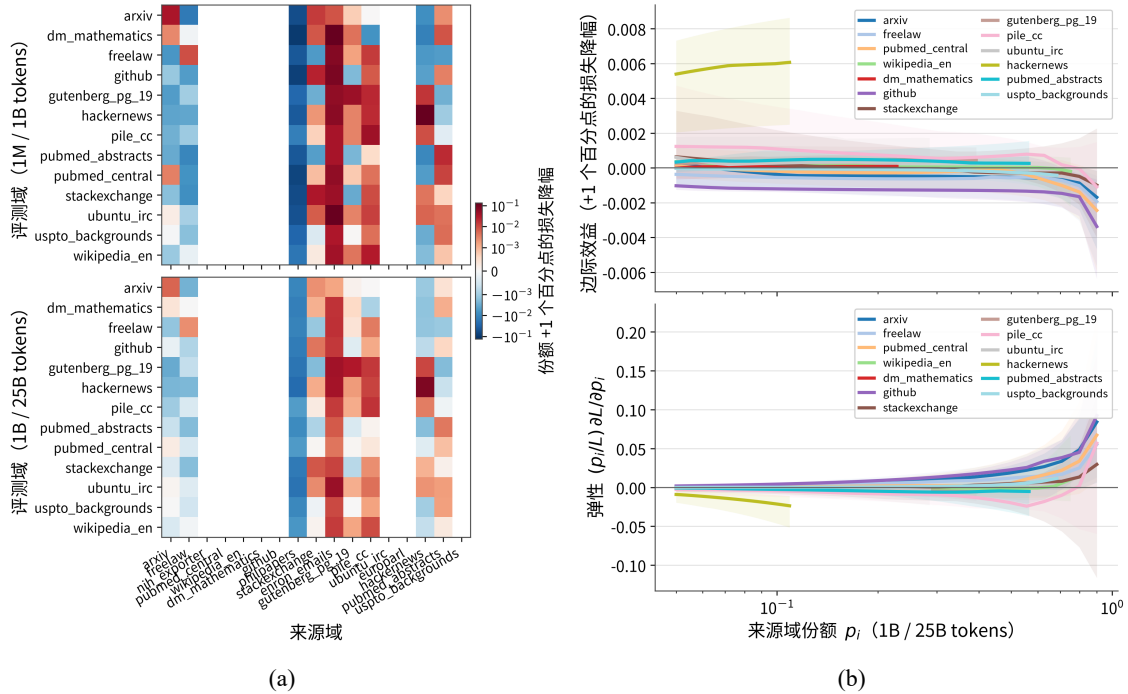
图 5.12 领域配比的方向异质性与份额依赖：(a) 不同来源增配 1 个百分点时，各评估目标的预测降损，红色表示降损、蓝色表示增损，空白表示不满足可行方向条件；(b) 在观测支撑域内扫描来源份额所得的方向收益与弹性，色带反映跨评估目标的分布范围。两图均为模型敏感度分析，不作因果解释。
