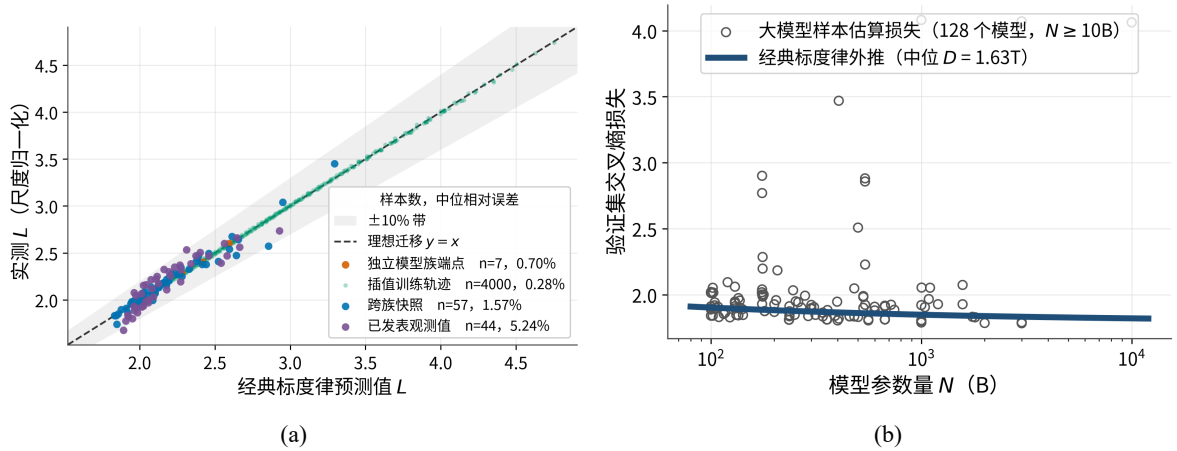
图 5.8 经典标度律的跨来源验证与大模型外推：(a) 损失尺度归一化后的多来源预测一致性，虚线为理想预测，阴影区域表示相对误差不超过 10%；(b) 百亿参数以上模型区间的标度律外推，曲线按中位训练数据量计算。
