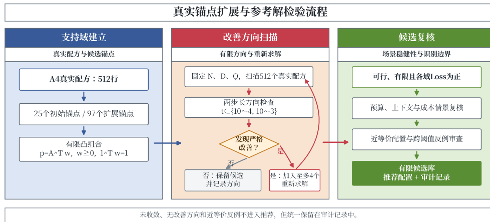
图 6.17 真实锚点扩展与参考解检验流程
