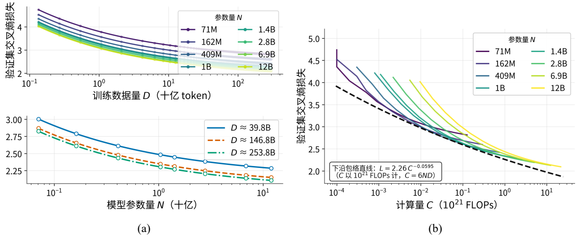
图 5.7 经典标度律的资源标度与计算效率：(a) 参数规模、数据规模与验证损失的标度关系。(b) 不同参数规模下计算量与验证损失的关系，虚线为经验下沿包络。
