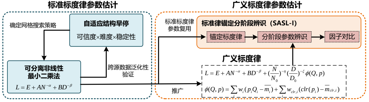
图 5.9 广义标度律的三阶段参数辨识：标准律锚定规模指数，分阶段估计组成响应与基线，再由规模因子对比确定响应幅度指数。图中 \phi 为组成损失修正的示意简写，正文记作 \varphi 。
