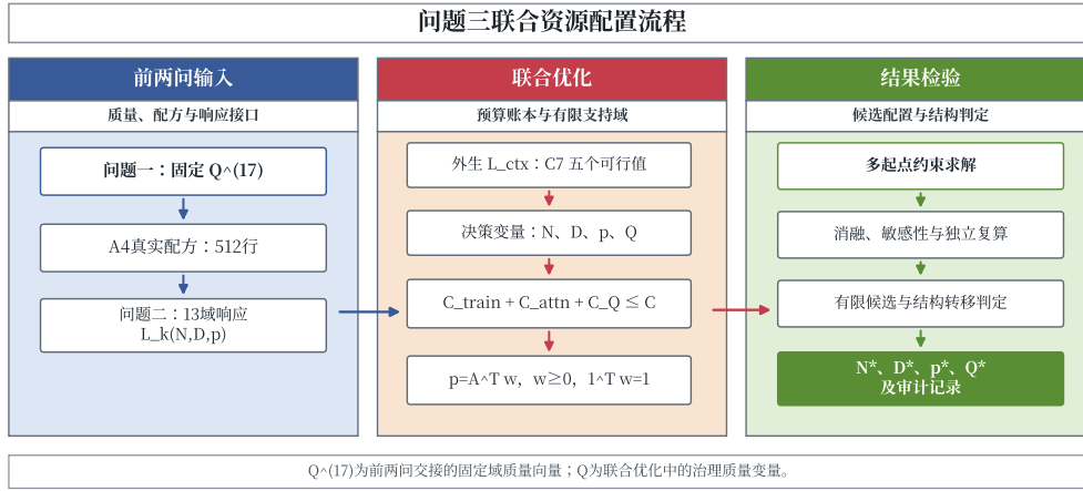
图 6.15 质量、配方及规模响应的衔接与联合求解流程
