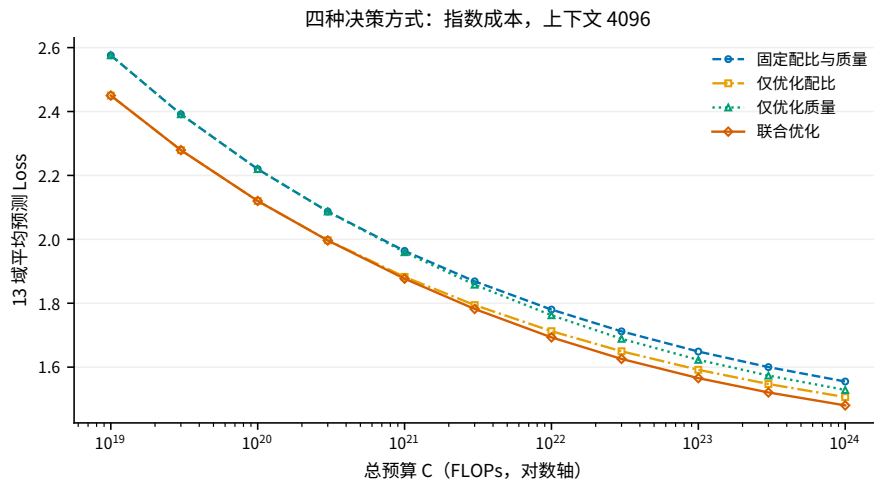
图 6.18 指数成本、上下文 4096 时 11 档预算的四组消融：各组均联动优化 N/D
