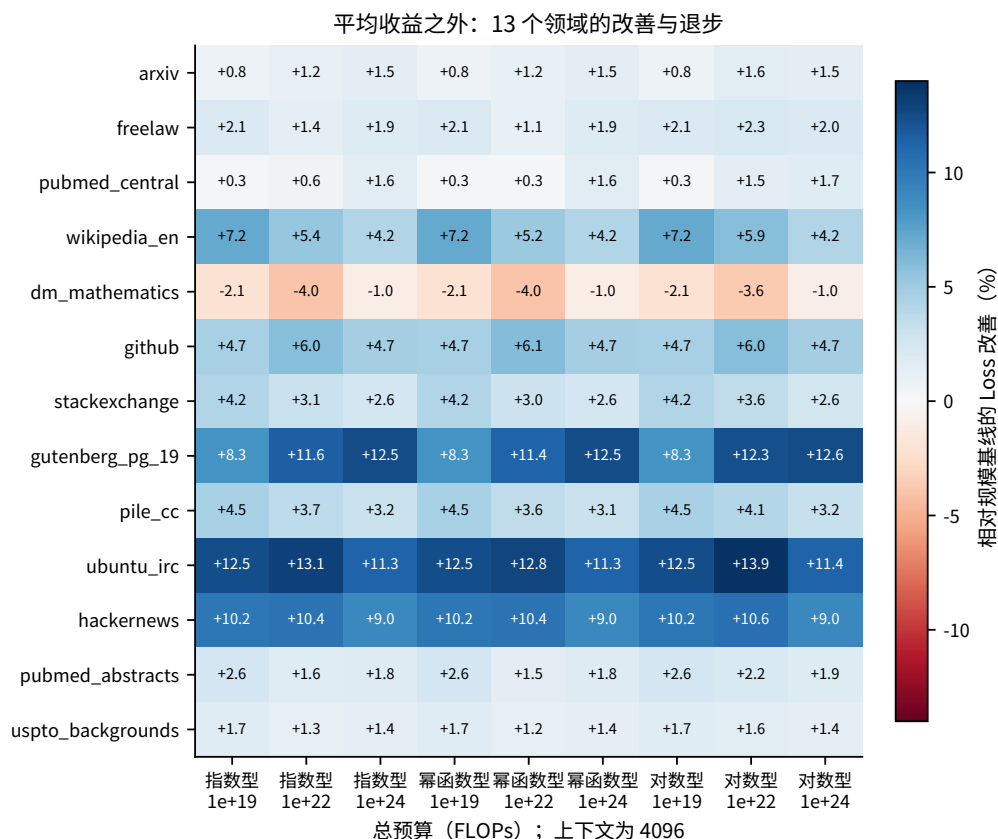
图 6.19 典型配置的逐域代价；热力图保留 13 个评测域和 9 组预算-成本组合，颜色表示相对原配方的 Loss 变化
