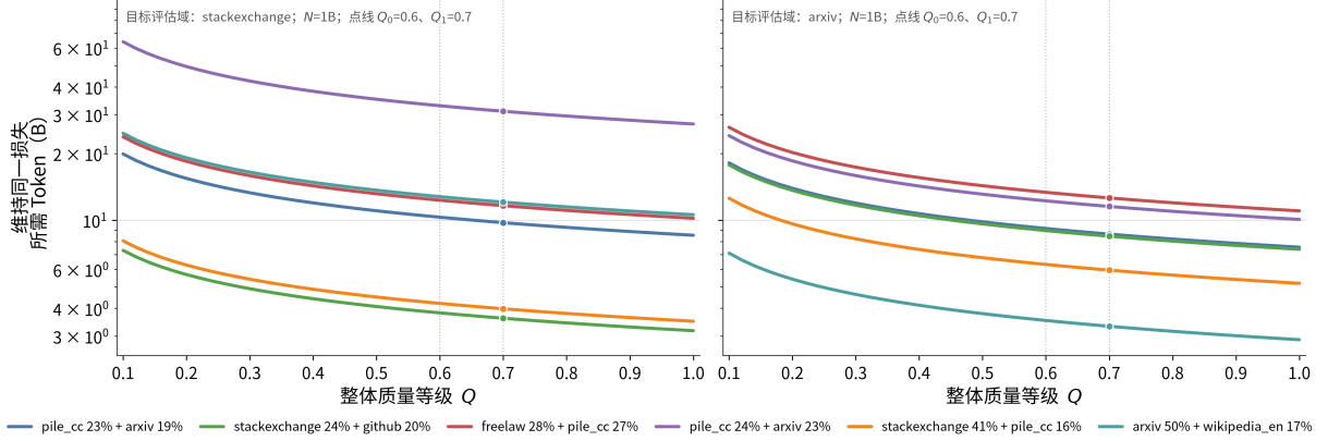
图 5.13 两种示例评估领域的质量—Token 等损失曲线。各曲线对应同一组观测配比，纵轴为保持参考目标损失所需的 Token 数； Q_0 = 0.6 与 Q_1 = 0.7 为质量比较点。离开 N = 10^9 , D_\star = 250 亿 Token 观测工作点后的需求量属于模型情景推算。
