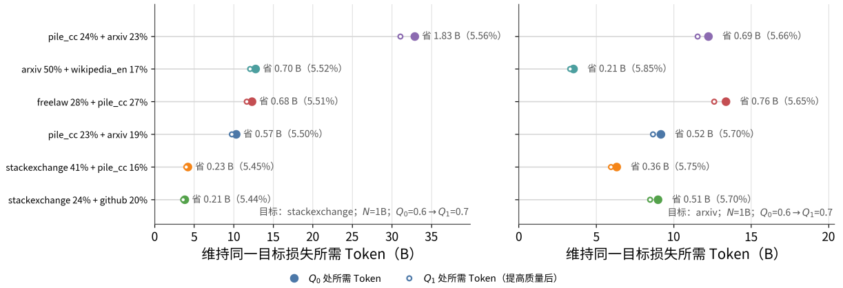
图 5.14 同一组观测配比在两种示例评估领域中的等损失 Token 需求。各行配比保持一致，实心与空心标记分别对应 Q_0 = 0.6 和 Q_1 = 0.7 ；横向差异表征模型预测的配比依赖性，并非配比干预的因果效应。
