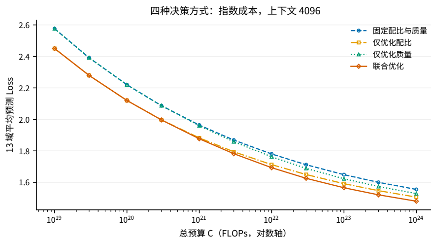
图 6.17 指数成本、上下文 4096 时 11 档预算的四组消融；各组均联动优化 N/D
