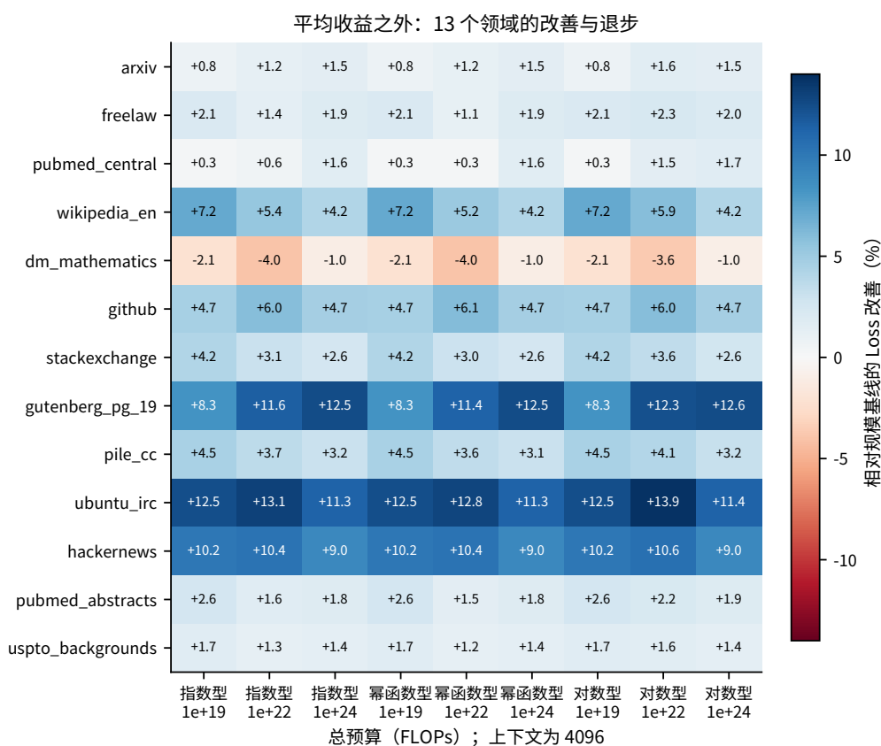
图 6.18 典型配置的逐域代价；热力图保留 13 个评测域和 9 组预算–成本组合，颜色表示相对原配方的 Loss 变化
