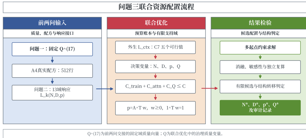
图 6.14 质量、配方及规模响应的衔接与联合求解流程
