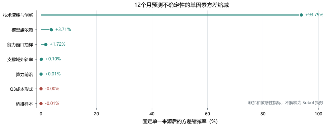
图 7.7 12 个月能力预测不确定性的单因素方差缩减
