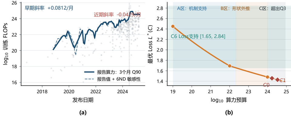
图 7.4 训练算力演进与 Q3–C6 共同支持边界
