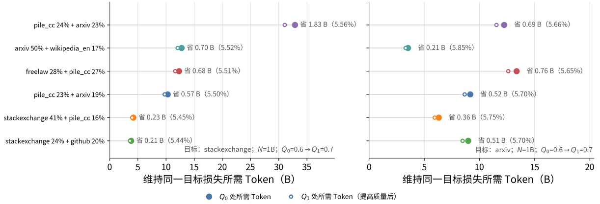
图 5.13 同一组观测配比在两种示例评估领域中的等损失 Token 需求。各行配比保持一致，实心与空心标记分别对应 Q_0 = 0.6 和 Q_1 = 0.7 ；横向差异表征模型预测的配比依赖性，并非配比干预的因果效应。
