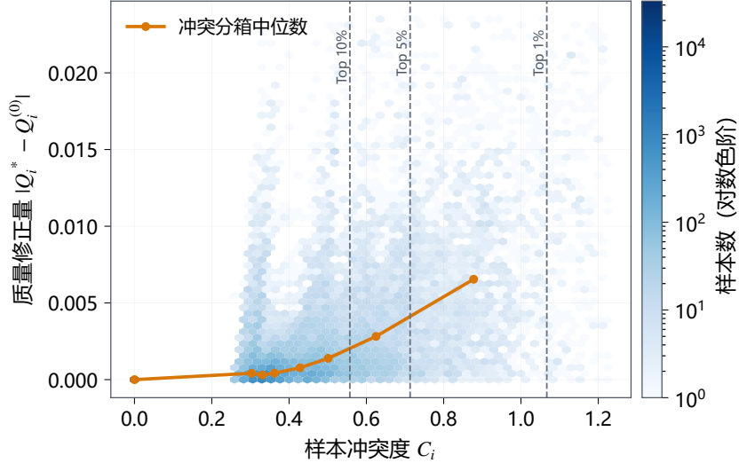
图 4.3 冲突修正的局部性与异常来源
