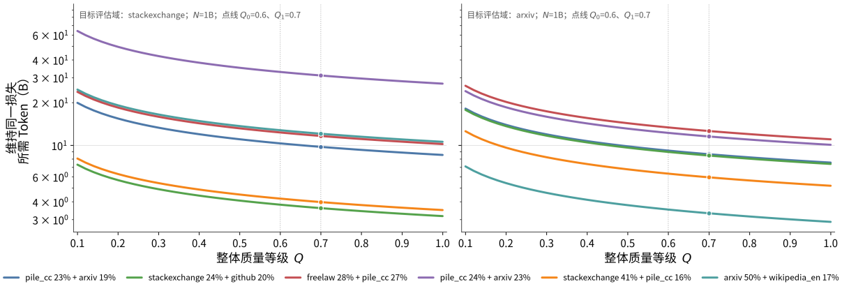
图 5.12 两种示例评估领域的质量-Token 等损失曲线。各曲线对应同一组观测配比，纵轴为保持参考目标损失所需的 Token 数； Q_0 = 0.6 与 Q_1 = 0.7 为质量比较点。离开 N = 10^9 , D_* = 250 亿 Token 观测工作点后的需求量属于模型情景推算。
