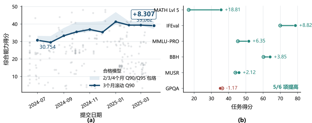
图 7.2 开放权重模型综合能力前沿与逐任务演进广度
