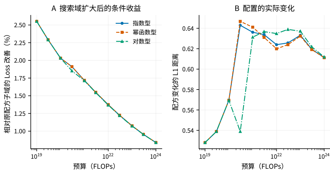
图 6.19 33 个 4096 上下文配置的扩域结果相对原 25 锚点联合解的变化
