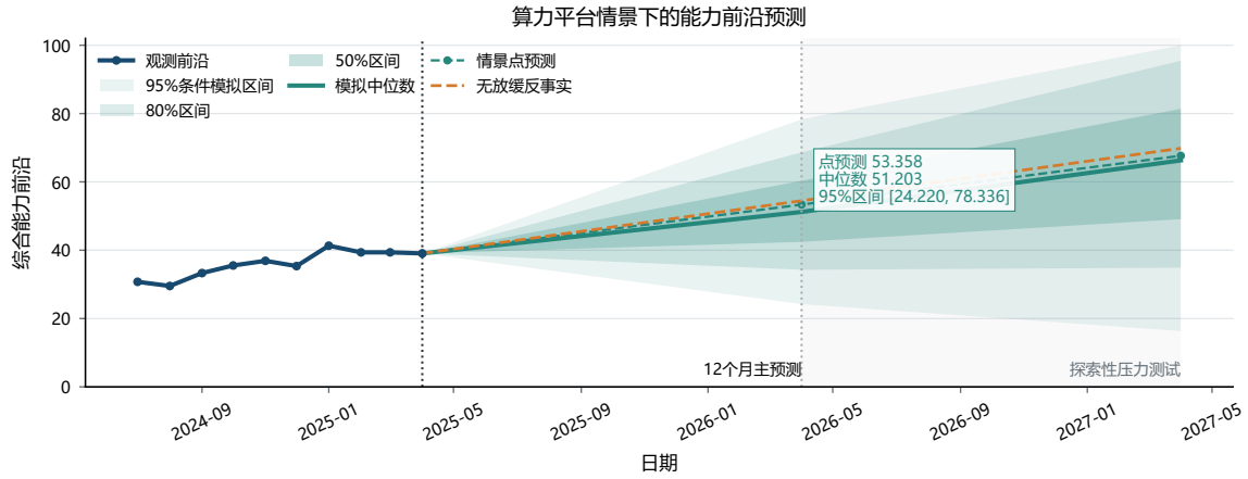
图 7.6 算力平台情景下开放权重模型能力前沿的条件预测
