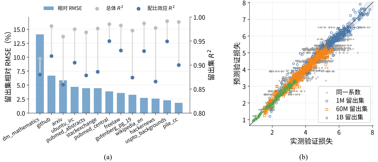
图 5.9 广义标度律的留出配比验证：(a) 各评估目标的相对 RMSE、总体 R^2 与配比效应 R^2 ；(b) 三个观测规模的实测与预测损失对比，灰色标记为同一组系数下关闭配比项的预测，实线为理想一致线，阴影表示 \pm 5\% 误差带。
