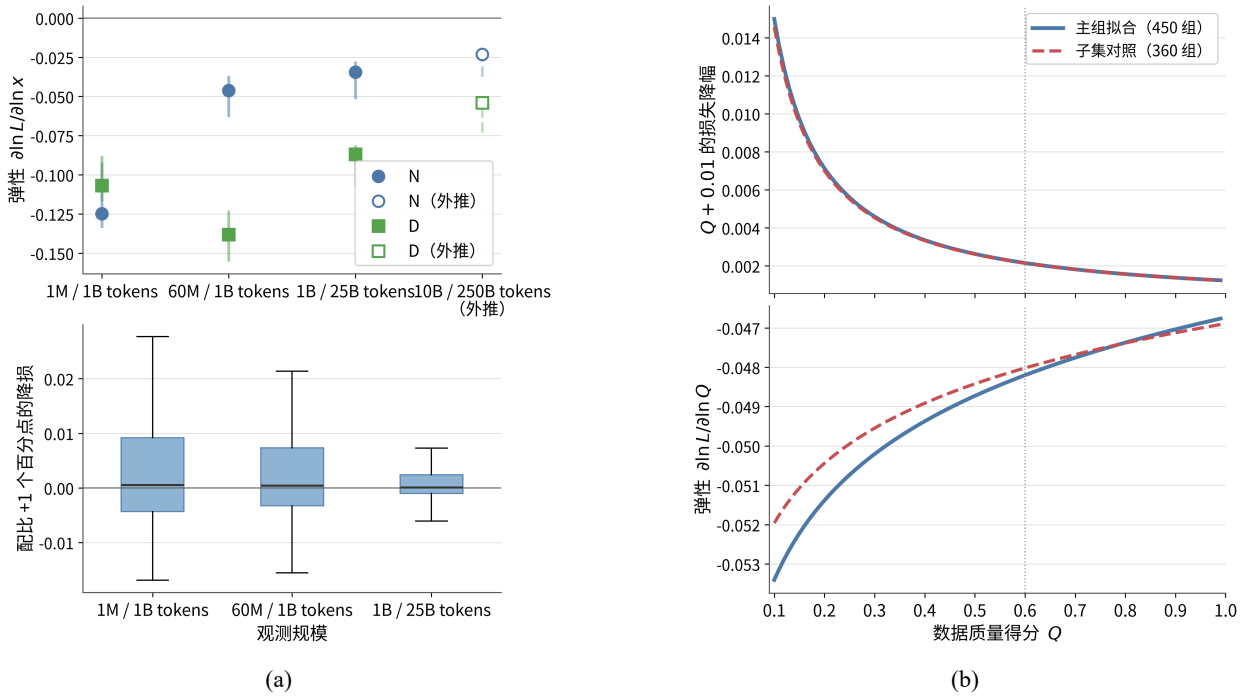
图 5.10 资源与质量因素的局部响应：(a) 参数量和数据量的损失弹性，以及配比份额增加 1 个百分点的方向收益分布；区间表示跨评估目标的四分位范围，百亿参数点仅为外推。(b) 独立质量实验中质量分增加 0.01 的降损及损失弹性；对照组为主组子集。
