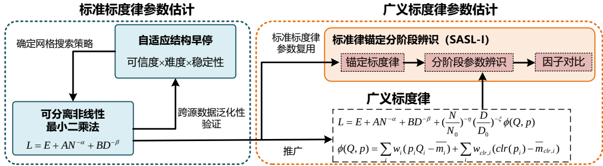
图 5.8 广义标度律的三阶段参数辨识：标准律锚定规模指数，分阶段估计组成响应与基线，再由规模因子对比确定响应幅度指数。图中 \phi 为组成损失修正的示意简写，正文记作 \varphi 。
