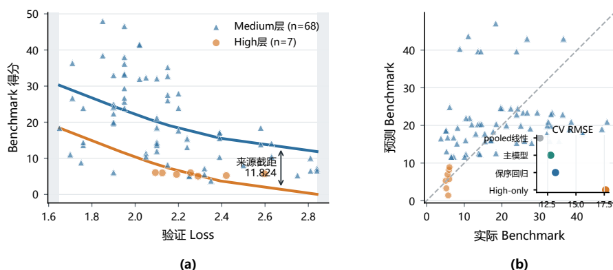
图 7.3 来源分层的 Loss–Benchmark 单调桥接与留出预测校准
