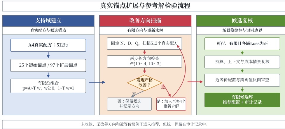
图 6.16 真实锚点扩展与参考解检验流程
