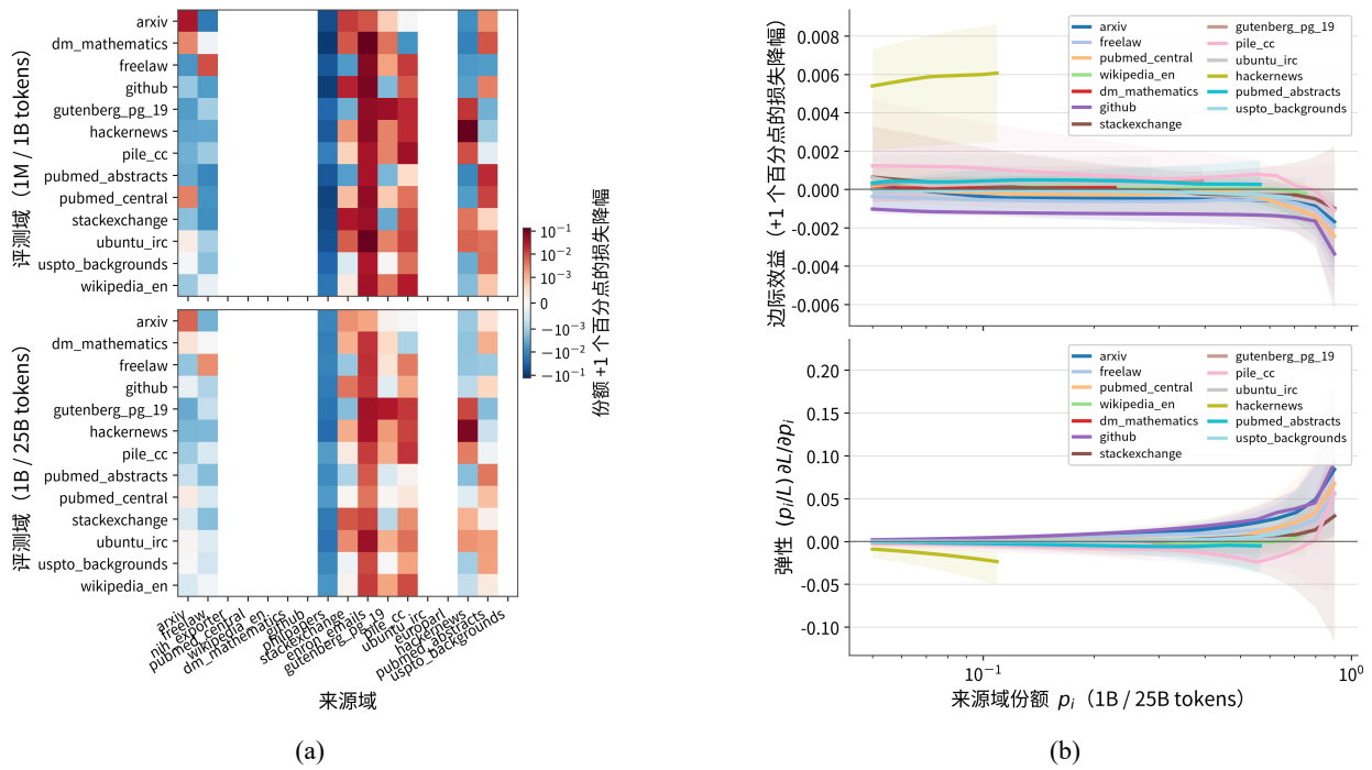
图 5.11 领域配比的方向异质性与份额依赖：(a) 不同来源增配 1 个百分点时，各评估目标的预测降损，红色表示降损、蓝色表示增损，空白表示不满足可行方向条件；(b) 在观测支撑域内扫描来源份额所得的方向收益与弹性，色带反映跨评估目标的分布范围。两图均为模型敏感度分析，不作因果解释。
