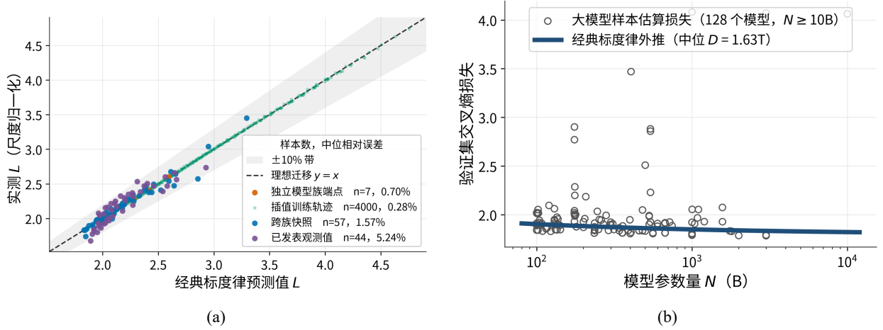
图 5.7 经典标度律的跨来源验证与大模型外推：(a) 损失尺度归一化后的多来源预测一致性，虚线为理想预测，阴影区域表示相对误差不超过 10%；(b) 百亿参数以上模型区间的标度律外推，曲线按中位训练数据量计算。
