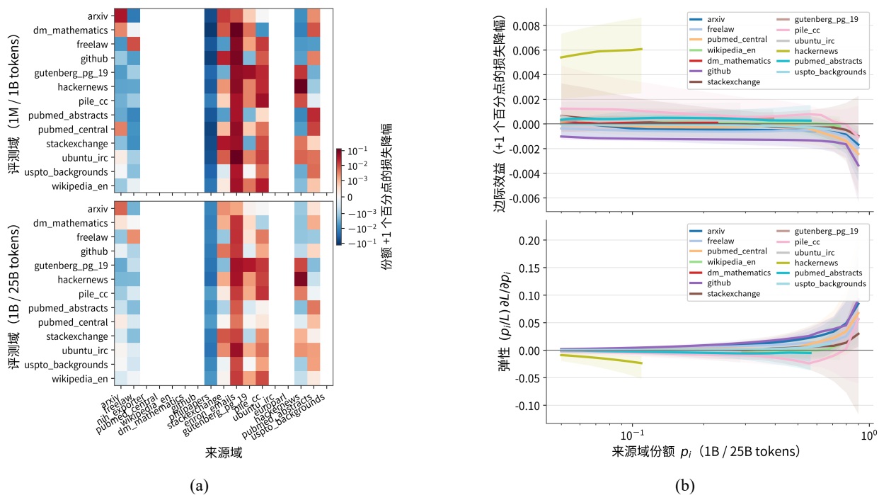
图 5.11 领域配比的方向异质性与份额依赖：(a) 不同来源增配 1 个百分点时，各评估目标的预测降损，红色表示降损、蓝色表示增损，空白表示不满足可行方向条件；(b) 在观测支撑域内扫描来源份额所得的方向收益与弹性，色带反映跨评估目标的分布范围。两图均为模型敏感分析，不作因果解释。
