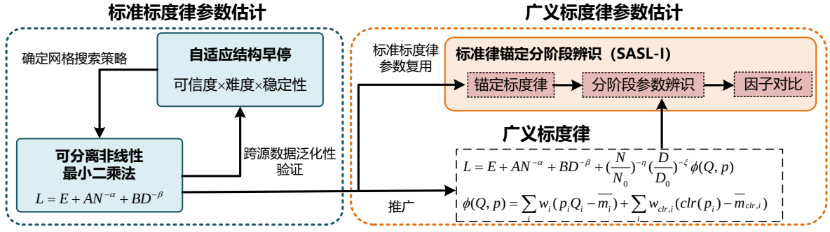
图 5.8 广义标准律的三阶段参数辨识：标准律锚定规模指数，分阶段估计组成响应与基线，再由规模因子对比确定响应幅度指数。图中 \phi 为组成损失修正的示意简写，正文记作 \varphi 。
