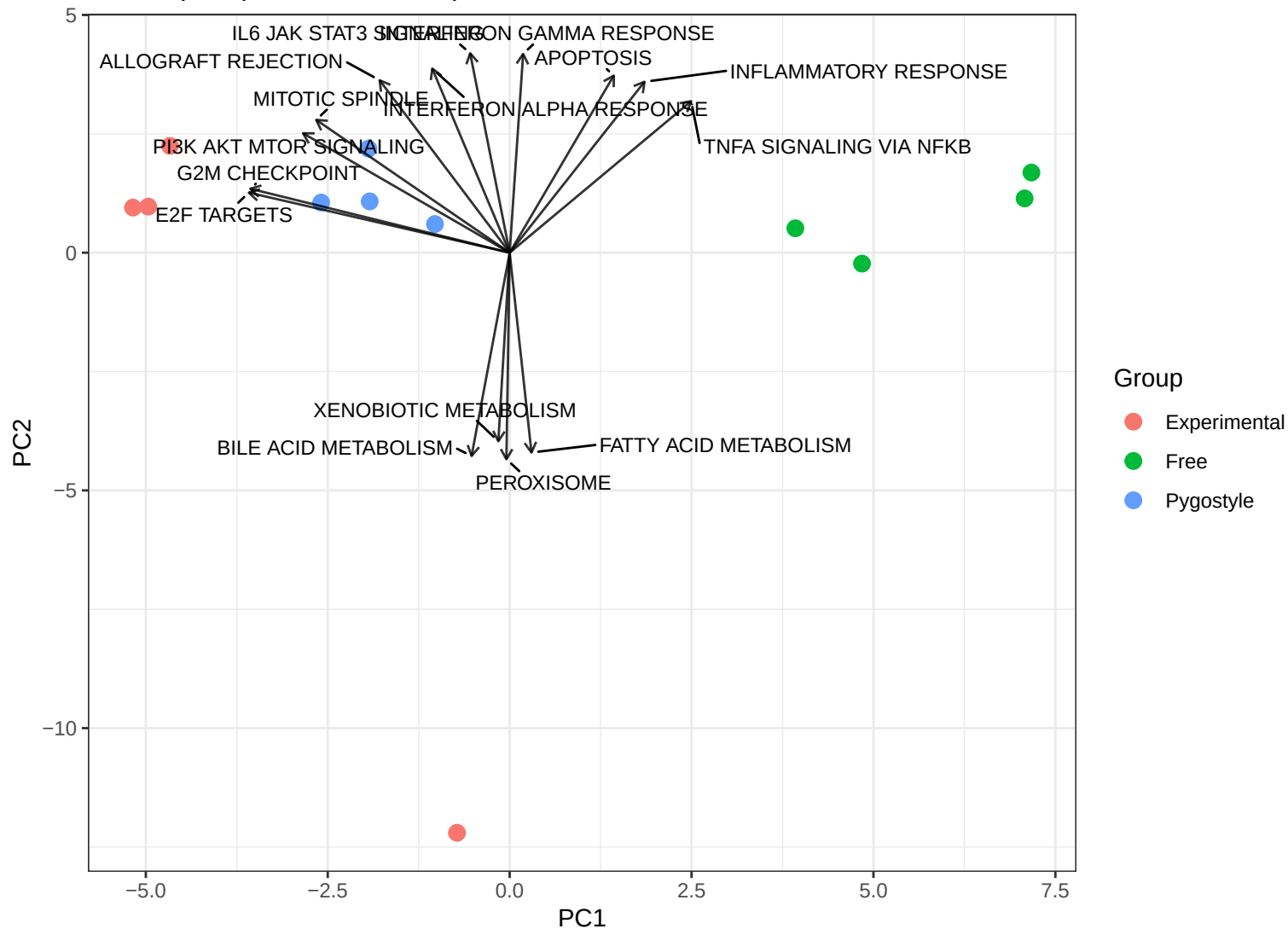
PCA biplot (ssGSEA scores)
