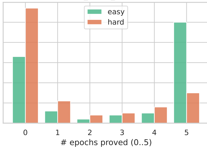
ops47_n-200_k-5 (k=5)
