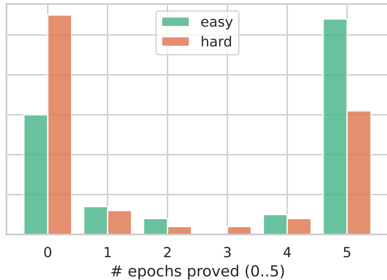
Sonnet 4.6 (k=5)
