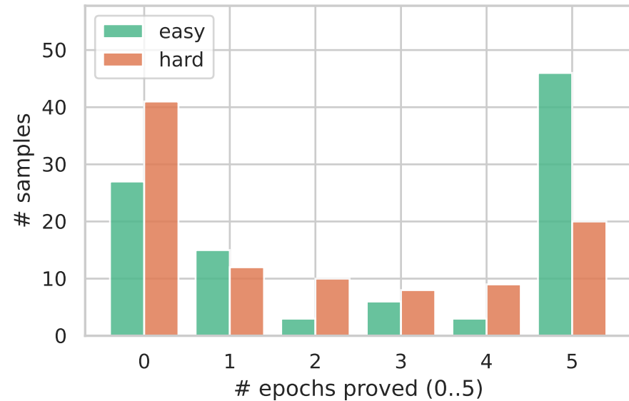
GPT-5.4 (k=5)
