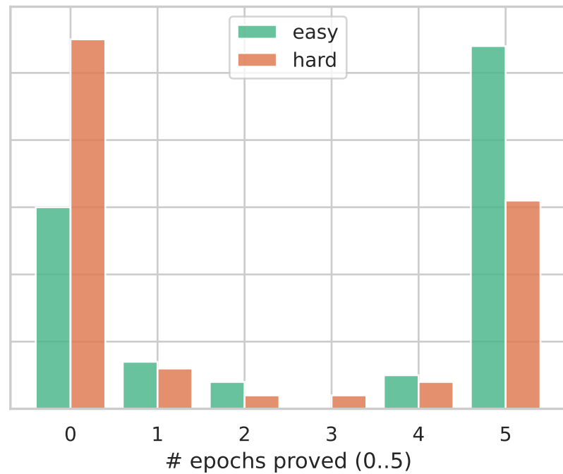
Sonnet 4.6 (k=5)
