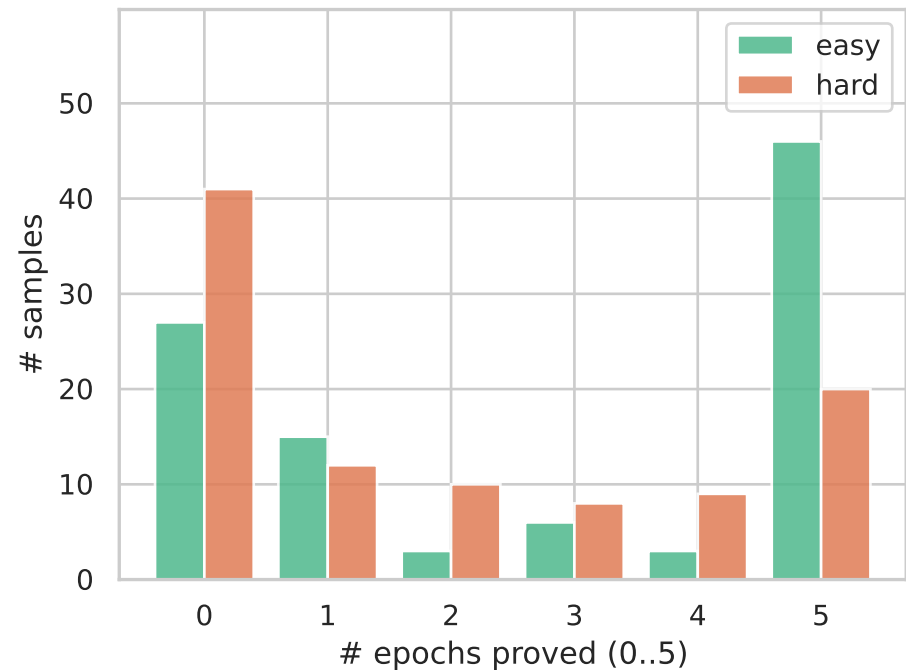
GPT-5.4 (k=5)
