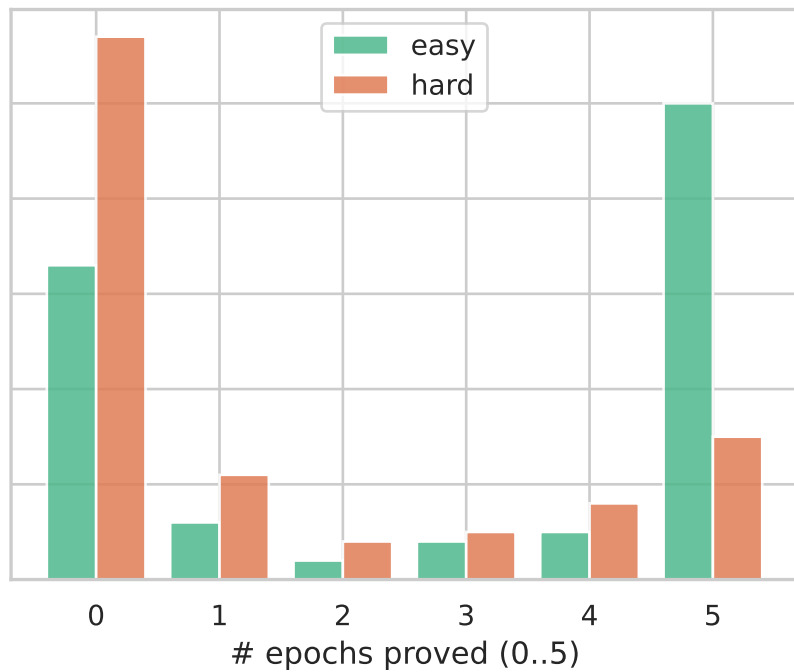
Opus 4.7 (k=5)
