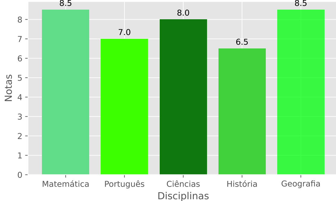
Disciplinas e suas notas - Turma B
