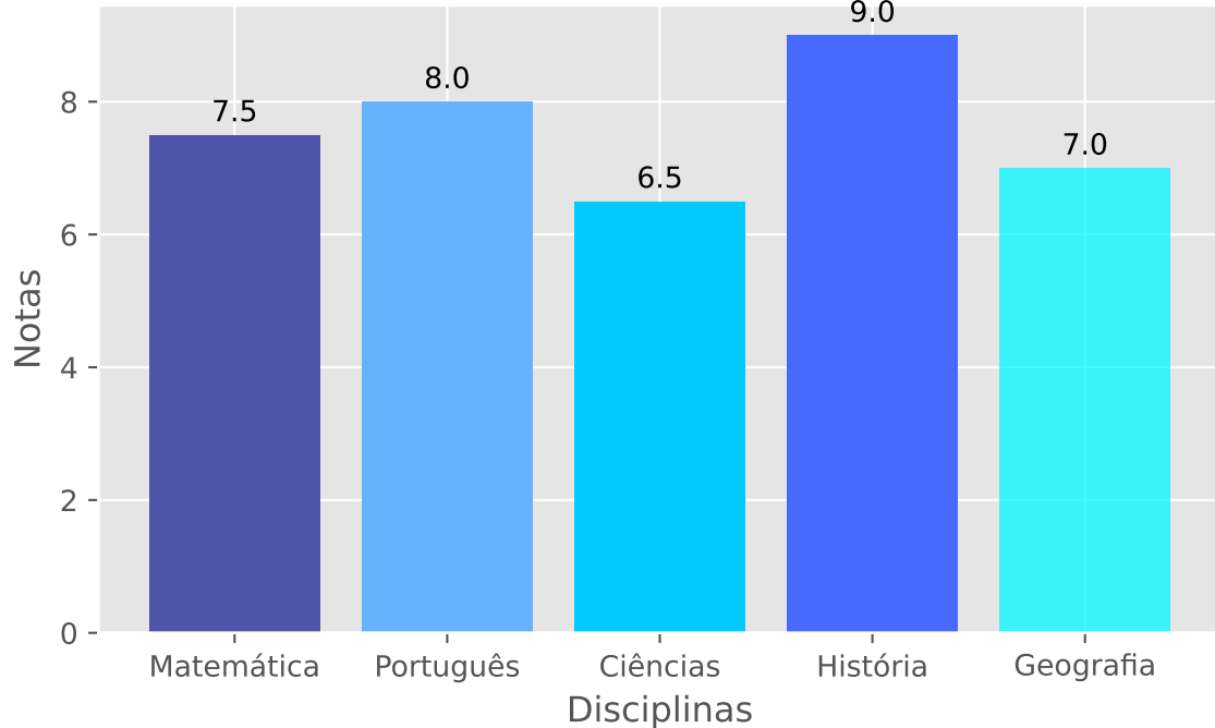
Disciplinas e suas notas - Turma A
