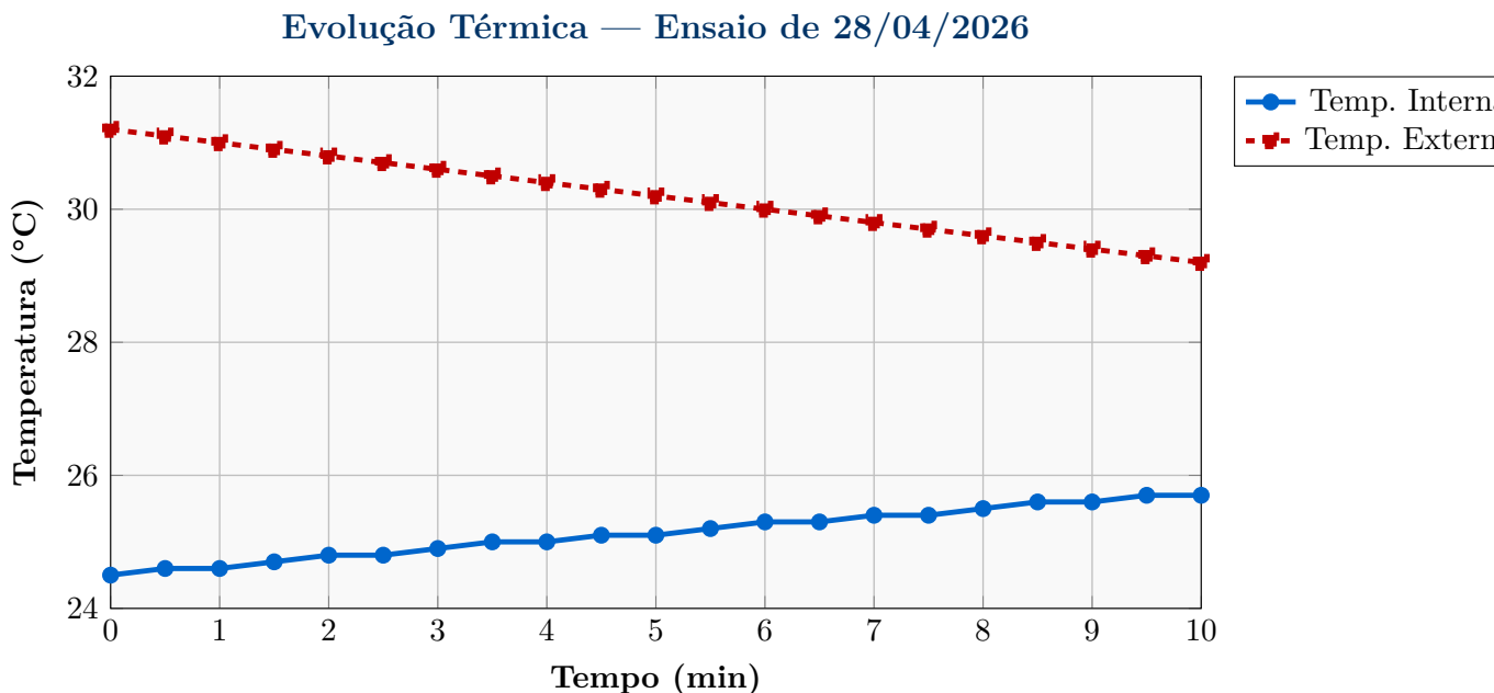
Figure 1: Temperaturas interna (azul) e externa (vermelho) em função do tempo de ensaio.
