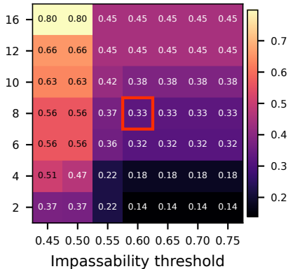
(b) Mean detour, min (common 20)
