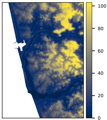
Curvature (-)
