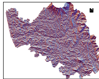
Aspect (°)
