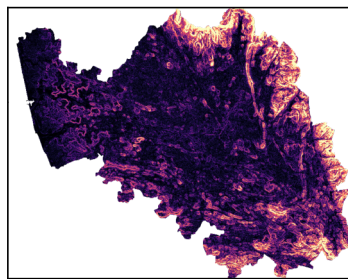
Slope (°)
