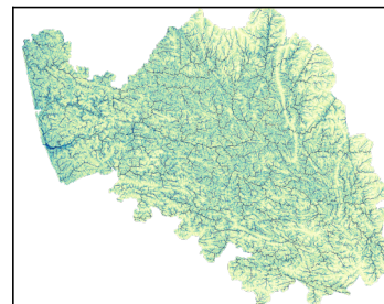
TWI (-)
