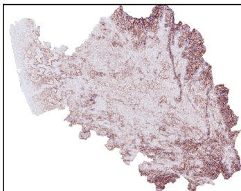
Curvature (-)
