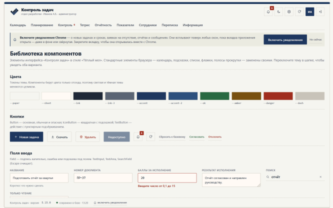
Рис. 31 Витрина библиотеки компонентов.
