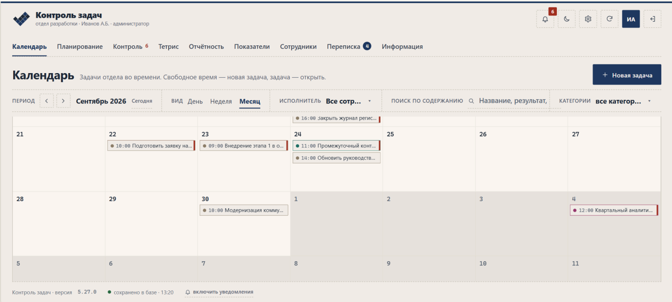
Рис. 4 «Месяц», страница прокручена: заголовок и фильтры на месте.
