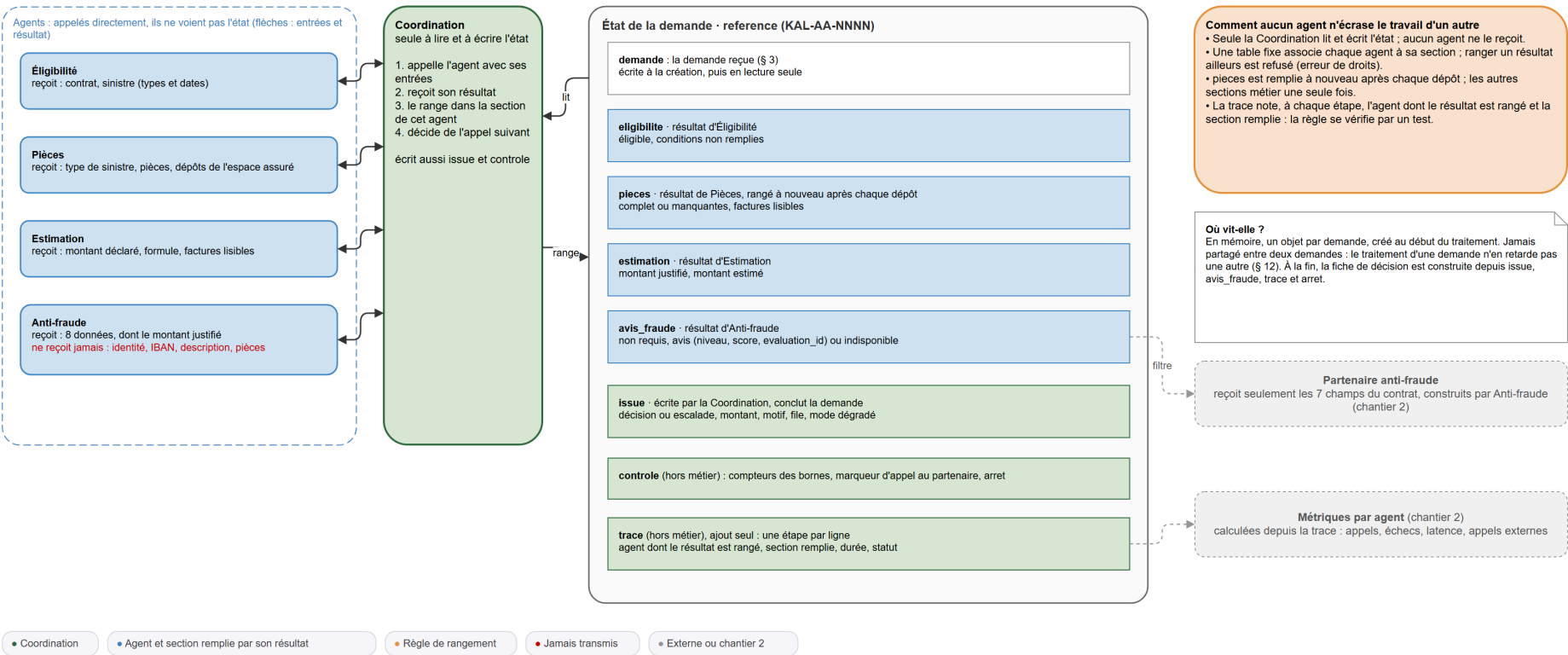
Figure 4 : Mémoire partagée : sections, droits et rangement.
