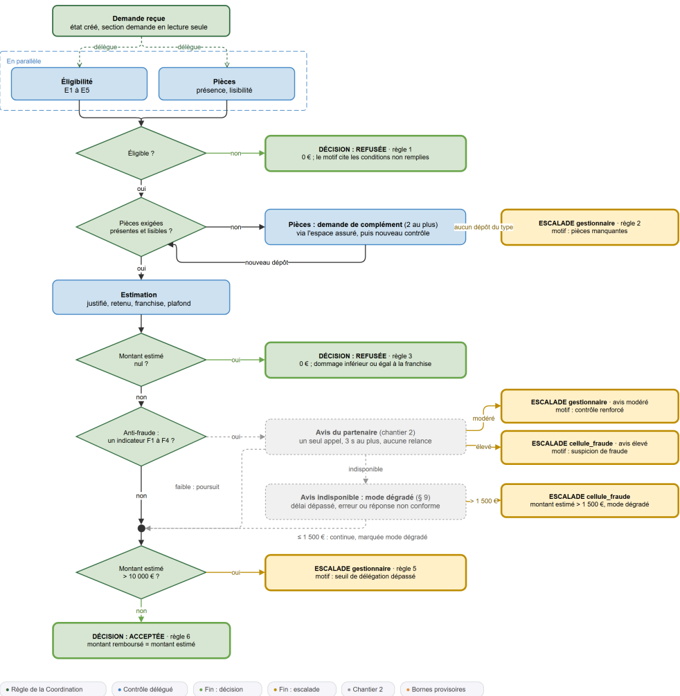
Figure 3 : Orchestration : règles de décision, boucle de complément, bornes et issues.
