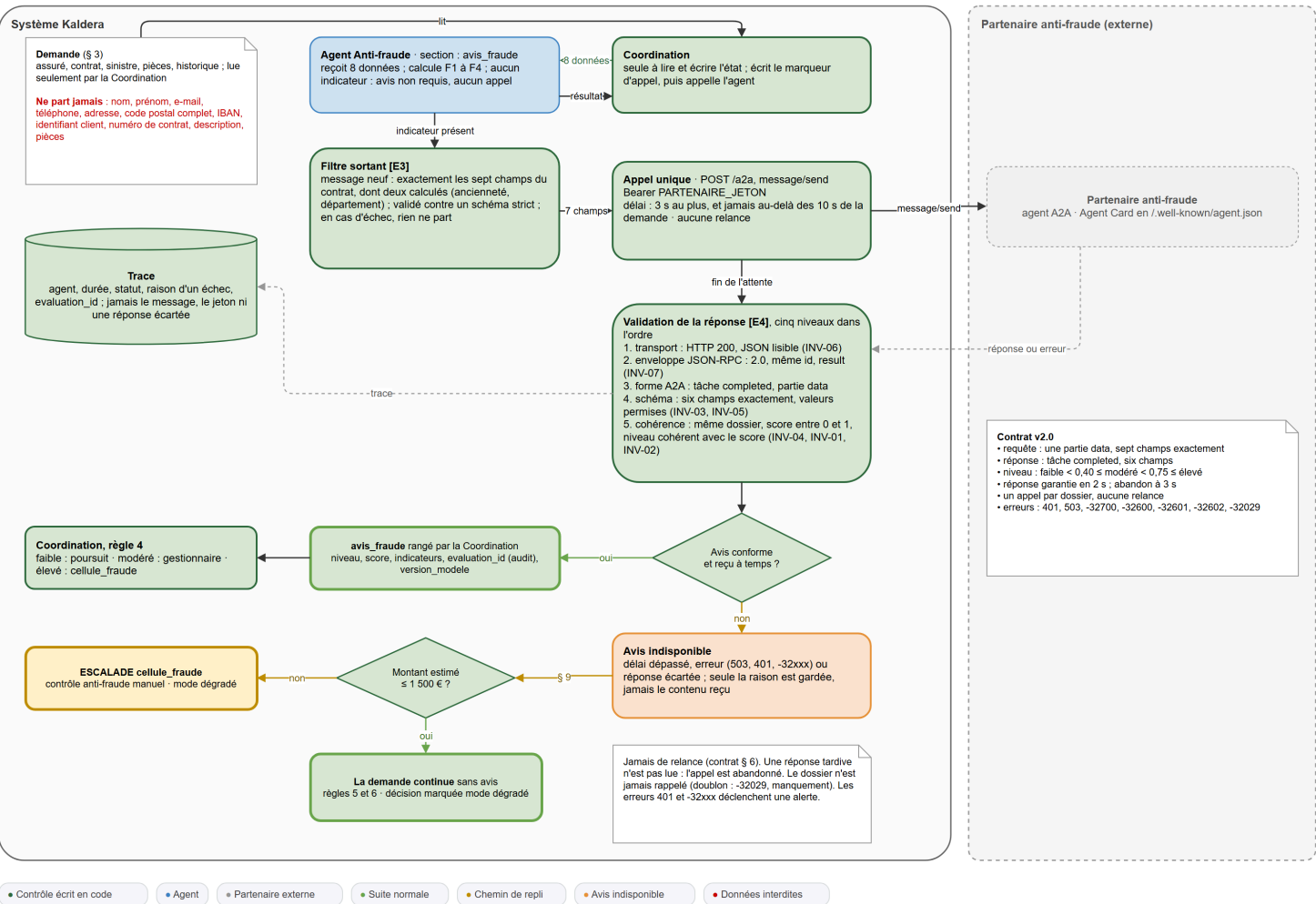
Figure 5 : Échange A2A : filtre, appel unique, validation et chemin de mode dégradé.
