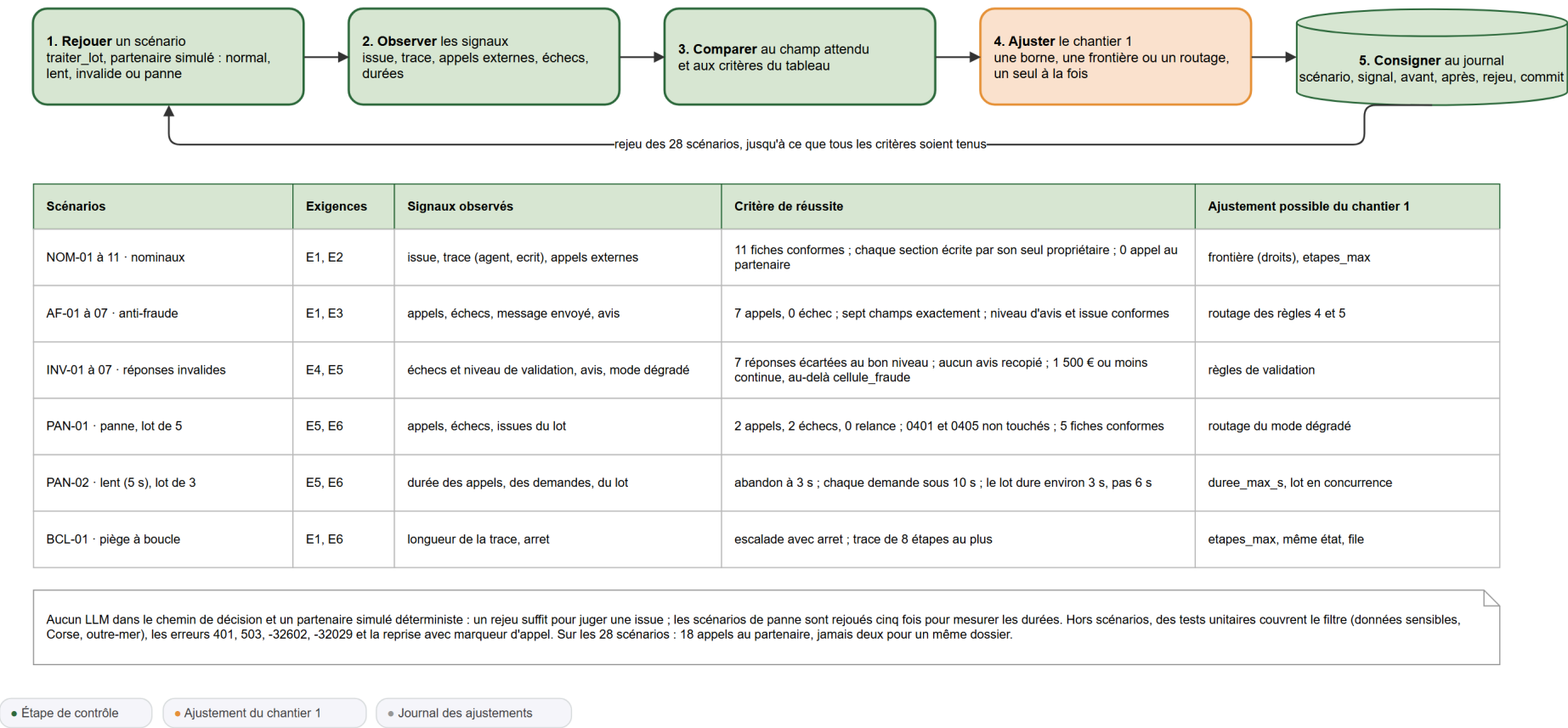
Figure 6 : Plan d'épreuve : rejouer, observer, comparer, ajuster, consigner. Version éditable : conception/schemas/schema-6-plan-epreuve.drawio
