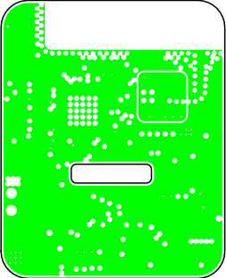
PWR (Scale 1:1)
