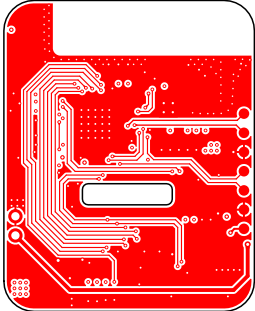
Top Layer (Scale 1:1)
