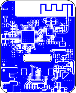
Bottom Layer (Scale 1:1)
