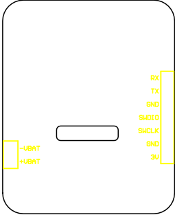
Top Overlay (Scale 1:1)
