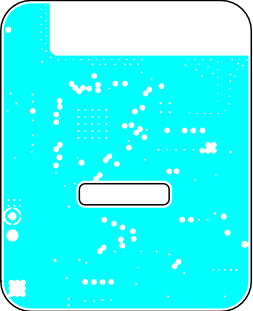
L2 (Scale 1:1)
