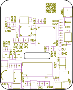
Bottom Overlay (Scale 1:1)
