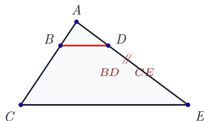
例题图：观察 BD \parallel CE 与对应边。
