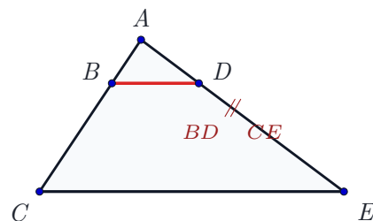
例题图：观察 BD \parallel CE 与对应边。
