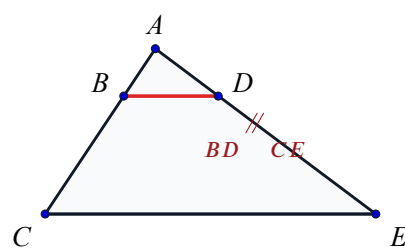
第 6 题图： BD \parallel CE
