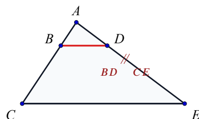
第 2 题图： BD \parallel CE
