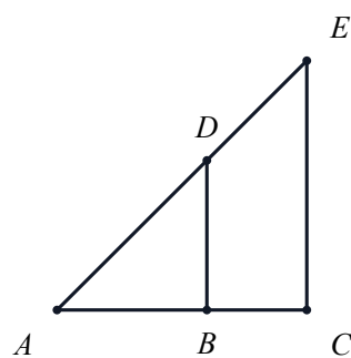
第3题图: 观察对应边和已知长度。
