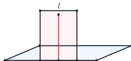
直线 l 在平面 \beta 内且垂直于平面 \alpha 。
