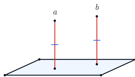
直线 a 、 b 都垂直于平面 \alpha 。
