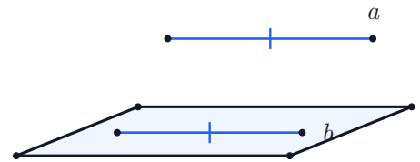
直线 a 在平面外、b 在平面内，且 a 与 b 平行。
