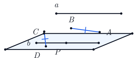
AB 在面外平行于平面，过 AB 作平面 \beta 与 \alpha 交于 CD。
