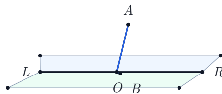
二面角 \alpha-l-\beta ， O 在棱 l 上， OA, OB 分别在两个面内。
