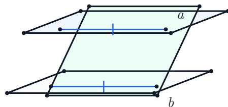
两平行平面 \alpha, \beta 被第三个面 \gamma 截出交线 a, b 。
