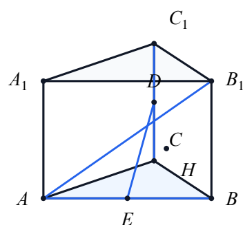
取 H 为 AB_1 中点，证 EHC_1D 为平行四边形。
