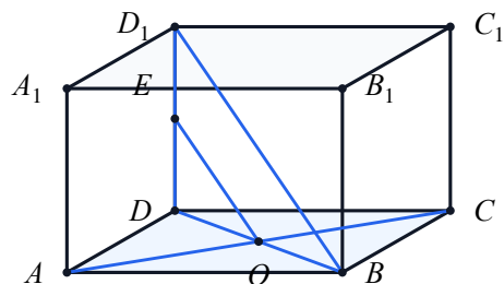
O 是 AC 与 BD 的交点，连 OE 看中位线。
