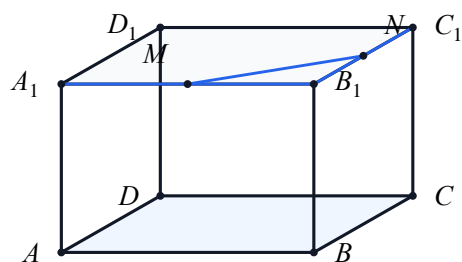
MN 是 \triangle A_1B_1C_1 的中位线。
