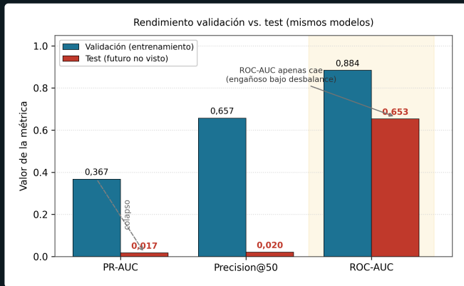
Figura 10. Rendimiento en validación y test sobre los mismos modelos: PR-AUC y precisión@50 colapsan; el ROC-AUC apenas cae. Fuente: elaboración propia.
