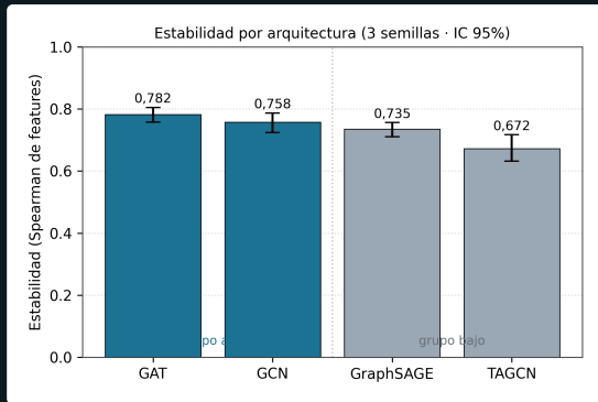
Figura 5. Estabilidad (Spearman de GNNExplainer) por arquitectura en Elliptic; 3 semillas, 180 modelos, IC 95 %.
