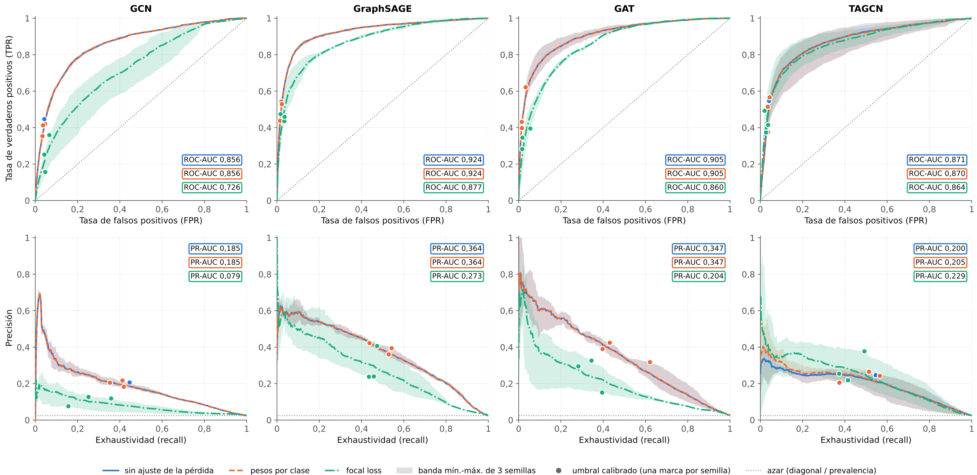
Curvas ROC y PR en validación · escenario 1:1 (submuestreo) (anexo) · media de 3 semillas · prevalencia 2,42 %
