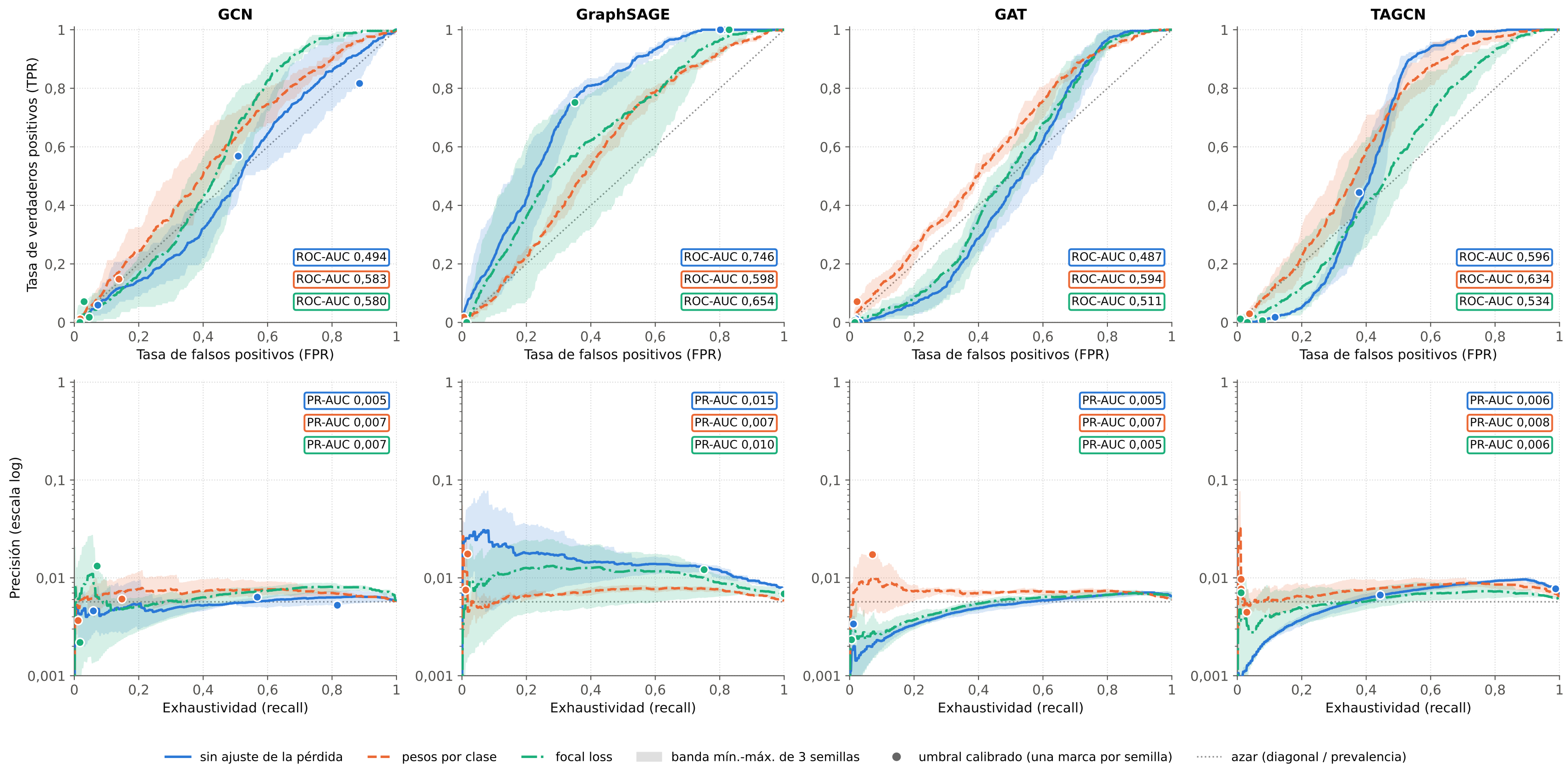
Curvas ROC y PR en test · escenario 1:100 (se quitan ilícitas) · media de 3 semillas · prevalencia 0,57 %
