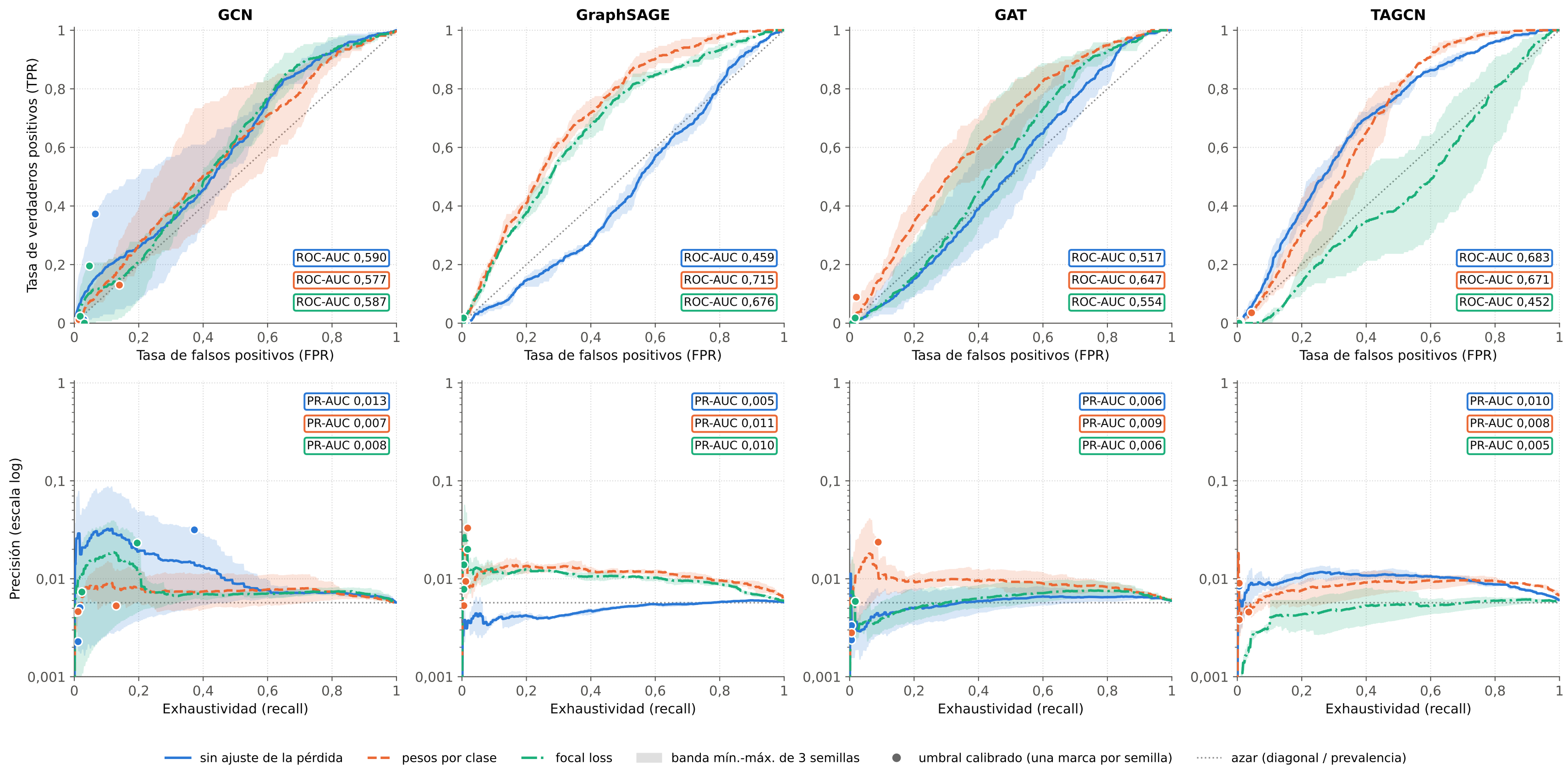
Curvas ROC y PR en test · escenario 1:10 con SMOTE · media de 3 semillas · prevalencia 0,57 %
