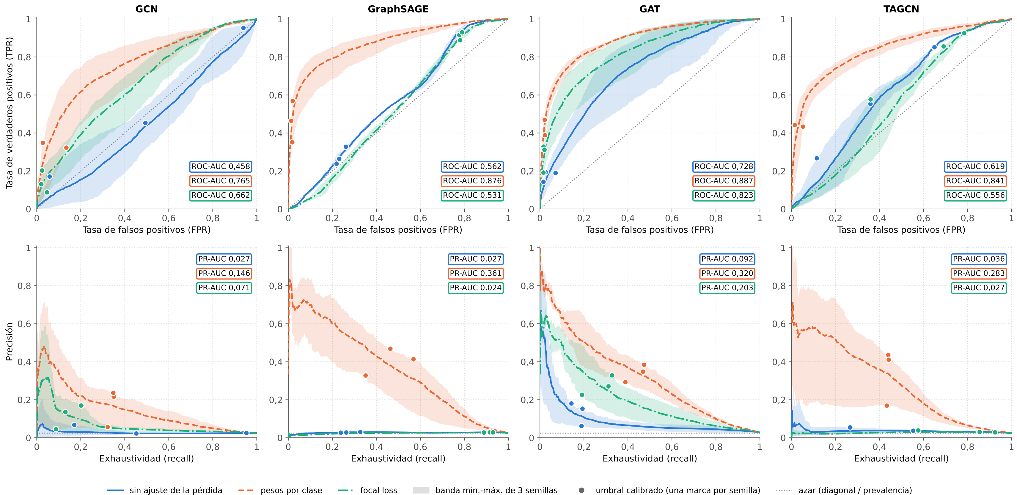
Curvas ROC y PR en validación · escenario 1:200 (se quitan ilícitas) · media de 3 semillas · prevalencia 2,42 %
