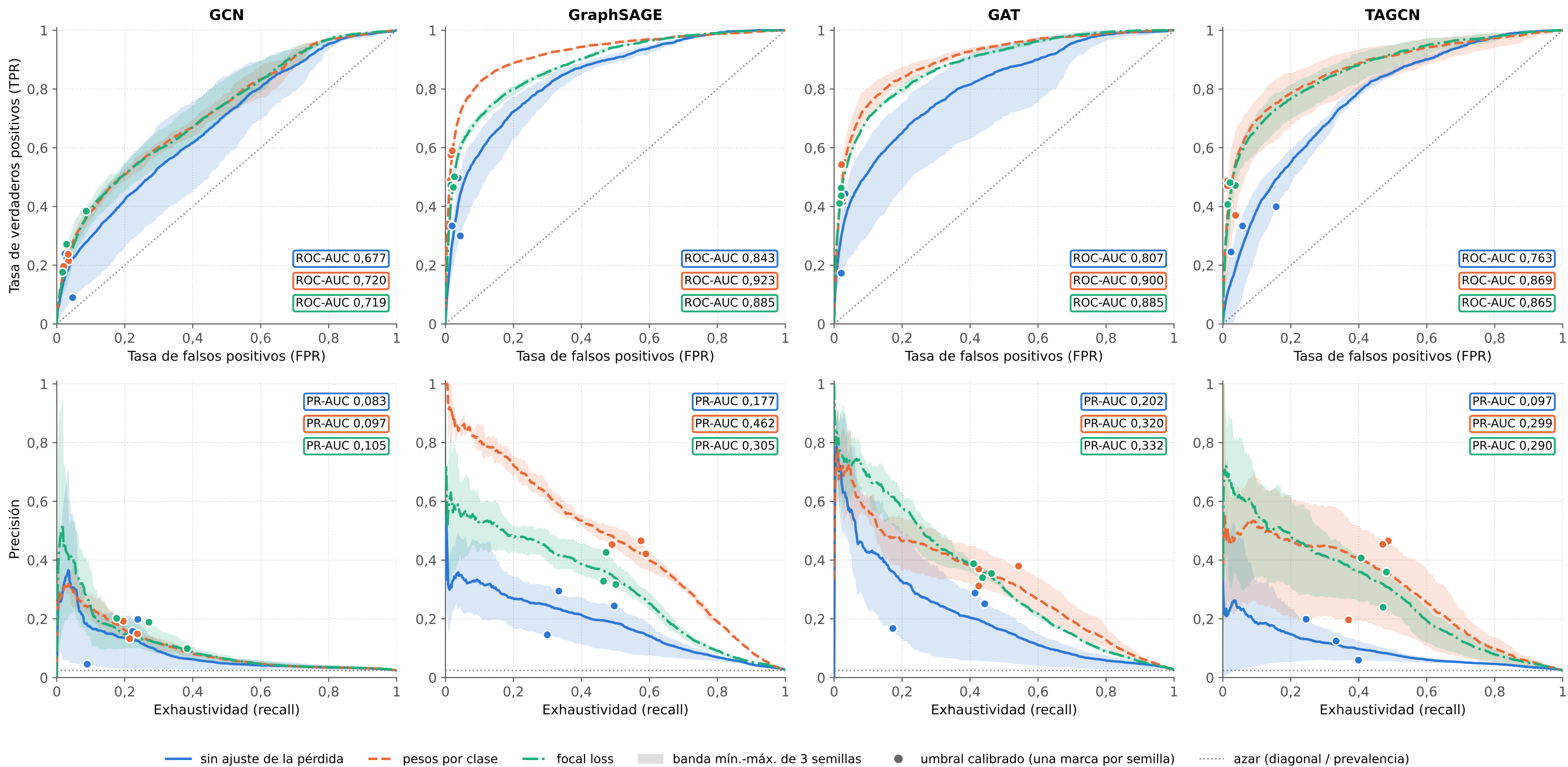
Curvas ROC y PR en validación · escenario nativo (1:38,4) · media de 3 semillas · prevalencia 2,42 %
