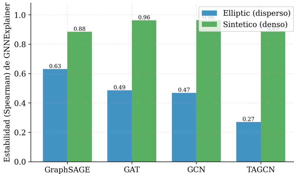
Figura 5.2: Estabilidad de GNNExplainer por arquitectura en los dos regímenes de densidad. En el grafo disperso de Elliptic GraphSAGE encabeza la estabilidad, mientras que en el grafo denso sintético lo hacen GCN y GAT, lo que evidencia que el orden depende de la densidad del grafo y no es una propiedad absoluta de la arquitectura.
