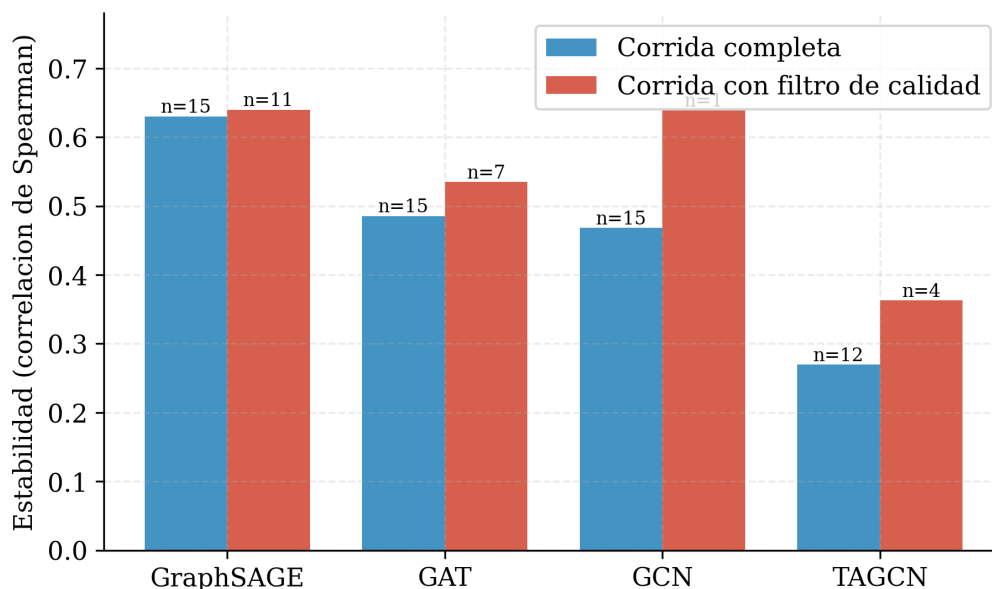
Figura 4.5: Estabilidad de las explicaciones por arquitectura sobre el subgrafo receptivo, en la corrida completa y en la corrida con filtro de calidad. GraphSAGE encabeza ambas corridas, mientras que GAT apenas varía entre subconjuntos, lo que evidencia que el ranking previo favorable a GAT era un artefacto del cálculo sobre el grafo completo.
