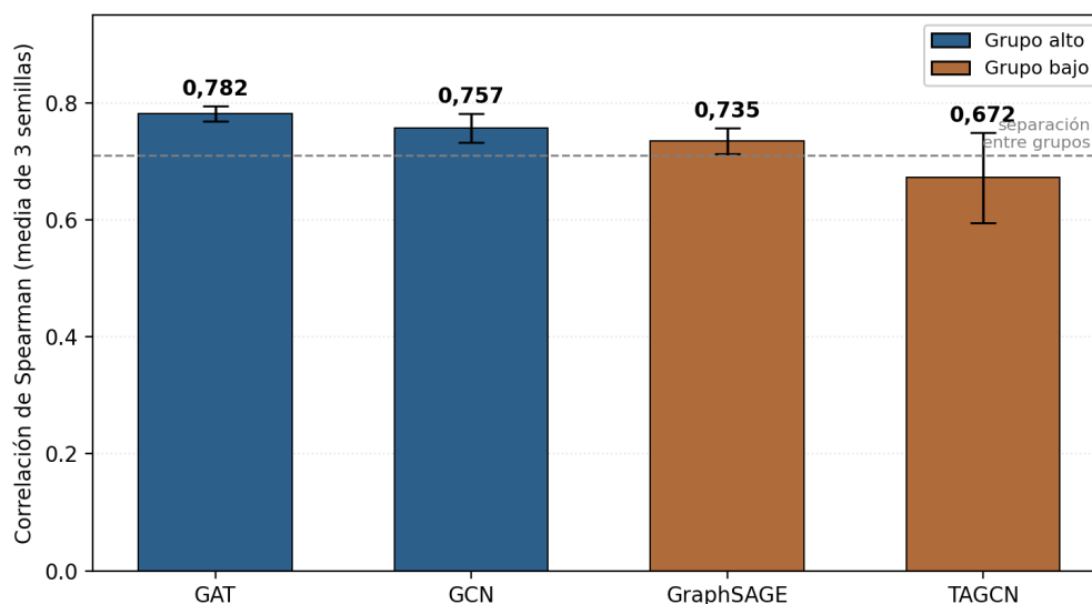
Figura 4.5: Estabilidad de las explicaciones por arquitectura sobre el subgrafo receptivo y con la métrica de Spearman corregida, promediada sobre las tres semillas de modelo, con barras de error que representan la desviación típica entre semillas. La prueba de rangos con signo separa un grupo alto formado por GAT y GCN de un grupo bajo formado por GraphSAGE y TAGCN, con diferencias significativas entre grupos y no dentro del grupo bajo. La mayor dispersión de TAGCN advierte contra fijar su valor central con demasiada precisión.
