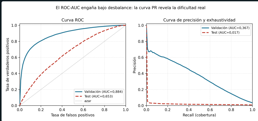
Figura 11. Curvas ROC (izquierda) y precisión-recall (derecha), validación vs test, mismos modelos. El ROC cae de 0,88 a 0,65, pero la precisión-recall se desploma casi a la tasa base de ilícitas: por eso la métrica primaria es PR-AUC, no ROC-AUC. Fuente: elaboración propia.
