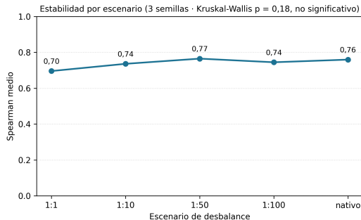
Figura 9. Estabilidad media por escenario de desbalance sobre Elliptic, promediada sobre las 3 semillas de modelo. Fuente: elaboración propia.
