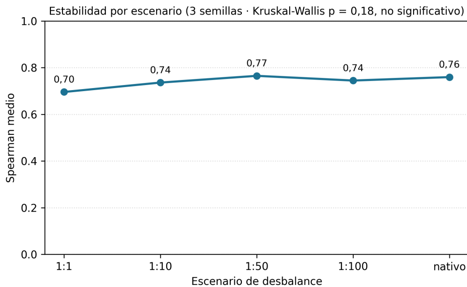
Figura 4.6: Estabilidad de las explicaciones por escenario de desbalance sobre el subgrafo receptivo, promediada sobre las tres semillas de modelo. La variación entre escenarios carece de dirección y no alcanza significancia estadística, con un valor p de 0,178 en la prueba de Kruskal-Wallis, lo que invalida la interpretación previa de un deterioro localizado.
